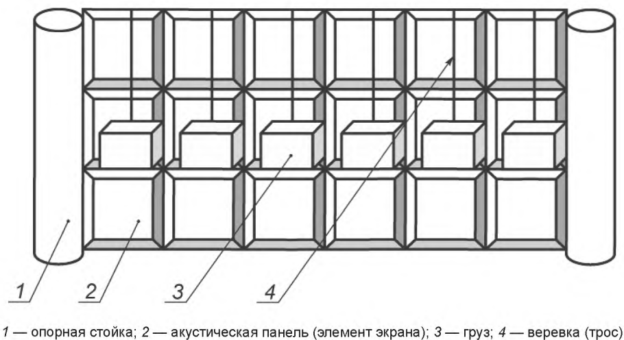
Рисунок Г.1 — Акустический экран
