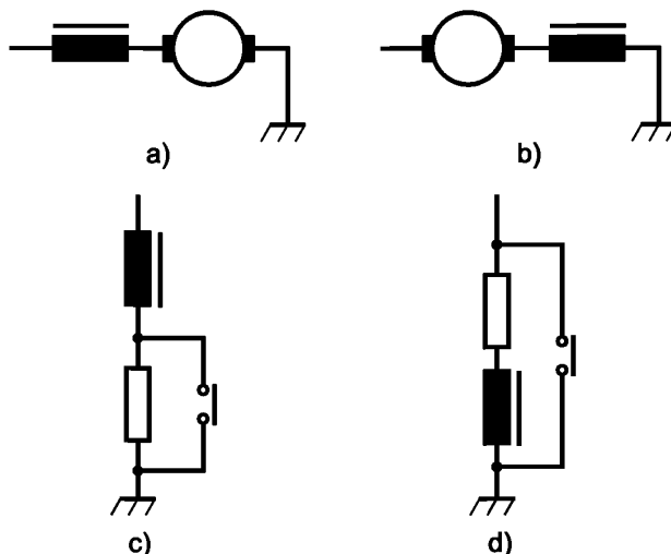
a) и b) — соединение обмотки возбуждения/якоря электродвигателя с последовательным возбуждением c) и d) — соединение при коротком замыкании имитируемой нагрузки
