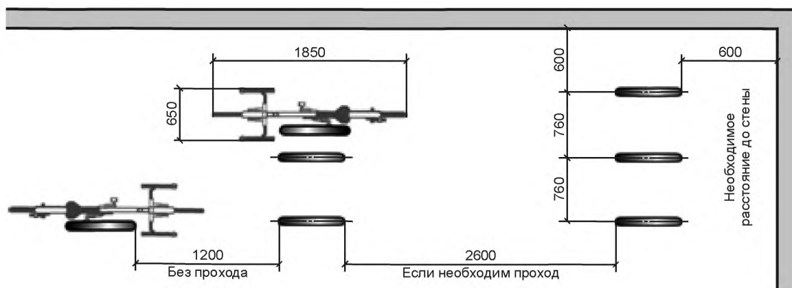
Рисунок 1 — Минимальные необходимые расстояния для создания велопарковки
