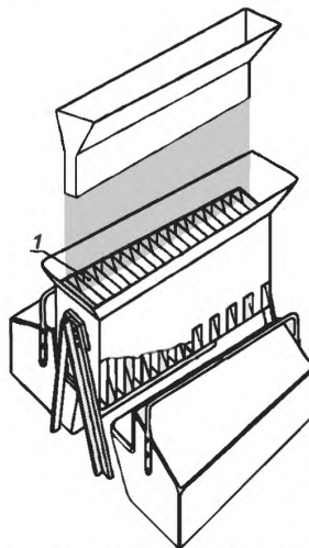
Рисунок 1 – Пример сократителя пробы
