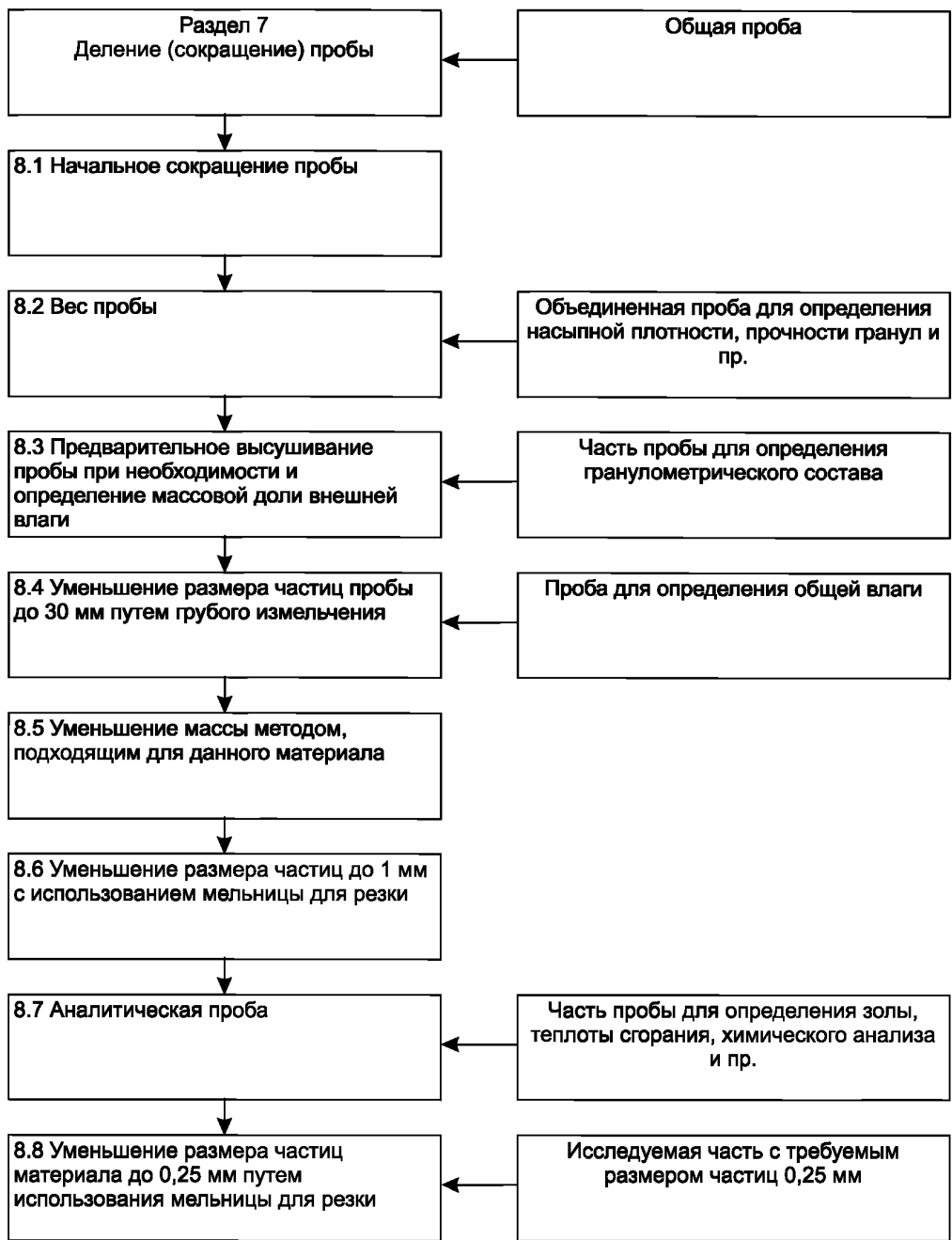
Рисунок 5 – Схема сокращения пробы
