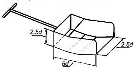
d – номинальный основной размер Рисунок 3 – Пример лопаты
