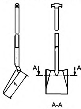
1 – длина совка; A-A – ширина совка Рисунок 4 – Пример совка
