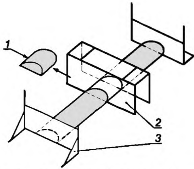
1 – точечная проба, 2 – рамка для отбора проб, 3 – конечные пластины Рисунок 7 – Сокращение квартованием с применением пластин
