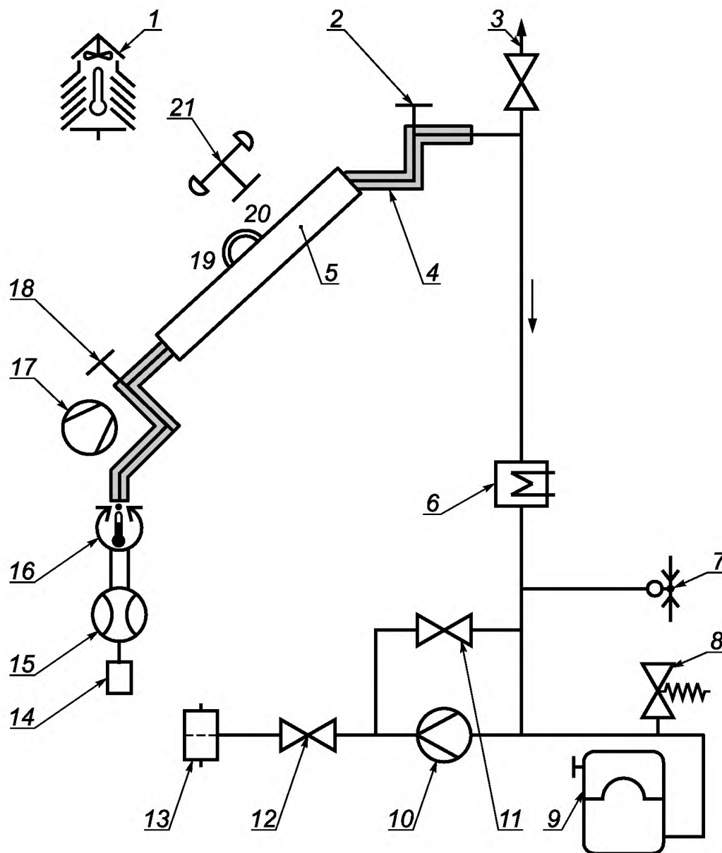
1 — датчик температуры окружающего воздуха; 2 — температурный датчик t_e ; 3 — вентиляционное отверстие; 4 — труба с двойными стенками; 5 — солнечный коллектор; 6 — нагреватель/охладитель для первичного регулирования температуры; 7 — манометр; 8 — предохранительный клапан; 9 — расширительный бак; 10 — насос; 11 — перепускной клапан; 12 — клапан-регулятор потока; 13 — фильтр (200 мкм); 14 — смотровое стекло; 15 — расходомер; 16 — вторичный регулятор температуры; 17 — вентилятор; 18 — датчик температуры t_{in} ; 19 — пиргеометр; 20 — пиранометр; 21 — анемометр
