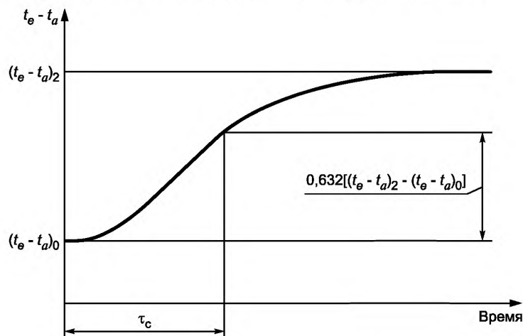
Рисунок 4 — Постоянная времени коллектора
