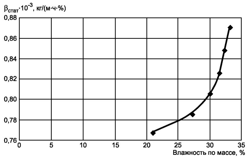
Рисунок А.3 — Зависимость коэффициента статической влажпроводности газобетона марки по средней плотности D500 от влажности
