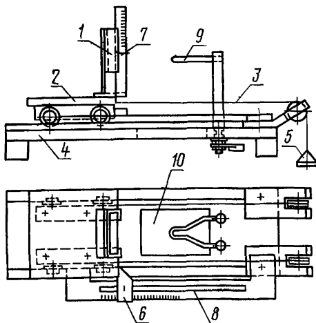
Устройство для испытания нагретой проволокой
