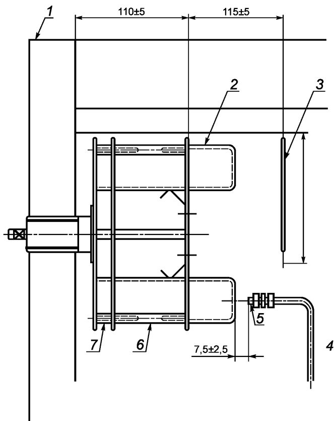
1 — печь; 2 — стеклянный контейнер (8 шт.); 3 — термометр; 4 — медная трубка диаметром ( 8,0 \pm 0,1 ) мм; 5 — форсунка диаметром ( 1,0 \pm 0,1 ) мм; 6 — втулка распорная передняя (4 шт.) длиной ( 55 \pm 1 ) мм; 7 — втулка распорная задняя (4 шт.) длиной ( 20 \pm 1 ) мм
