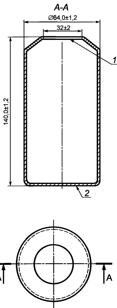
Рисунок 5 — Стекло́нный контейнер с горловиной, направленной наружу
