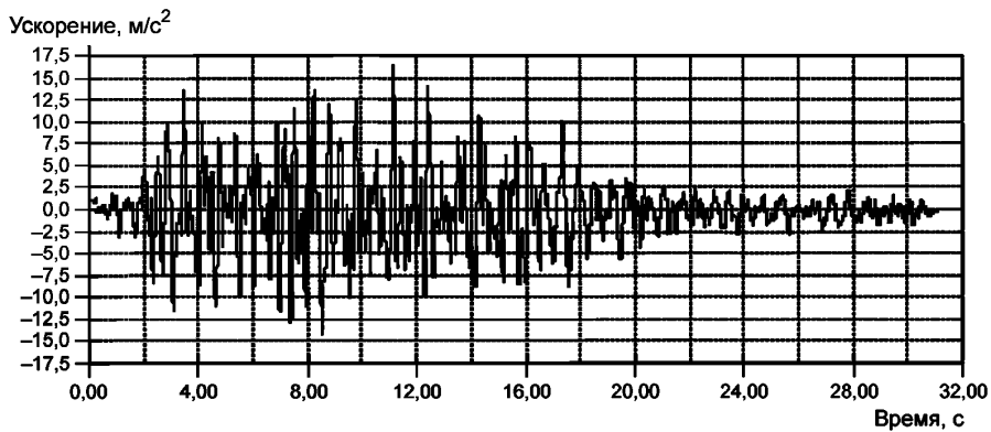
Рисунок 4 — Временная диаграмма тестового сигнала
