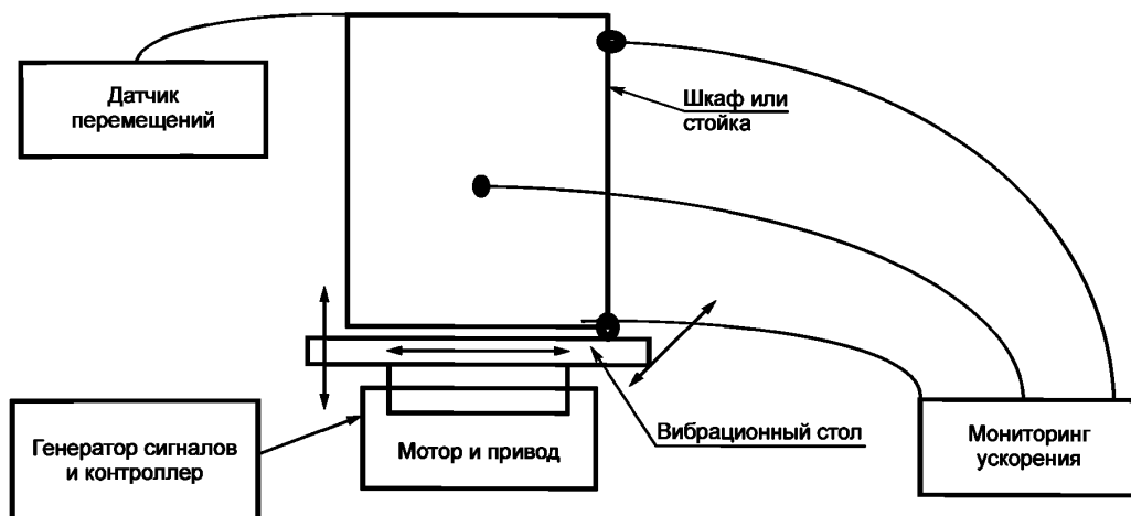
Рисунок 2 — Структурная схема испытания
