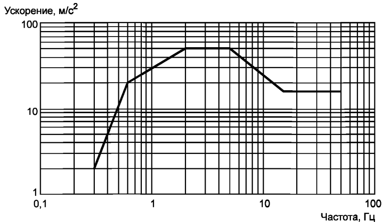
Рисунок 3 — ТСО для тестового сигнала (коэффициент демпфирования 2 %)
