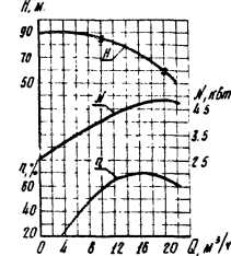
Характеристика насоса 33ЦДБ6-16-75
