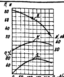
Характеристика насоса 34Б 12-210-55
