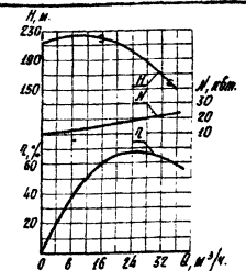
Характеристика насоса 34Б6-25-195
