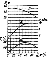
Характеристика насоса 34Б10-65-40Г
