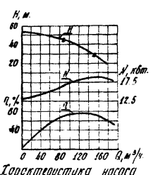
Характеристика насоса 34Б10-120-40Г
