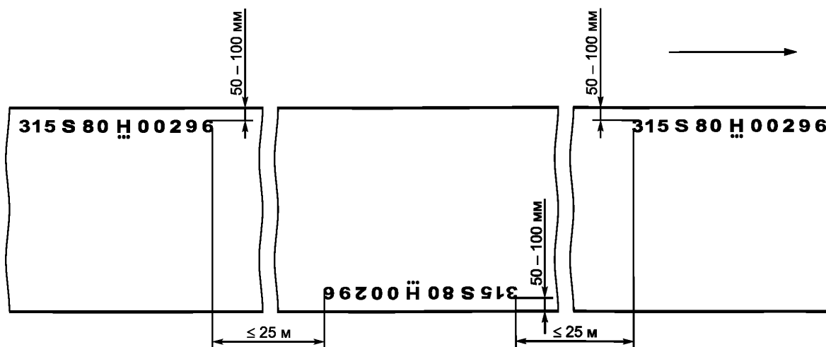
Рисунок 1 — Маркировка лент полной ширины
