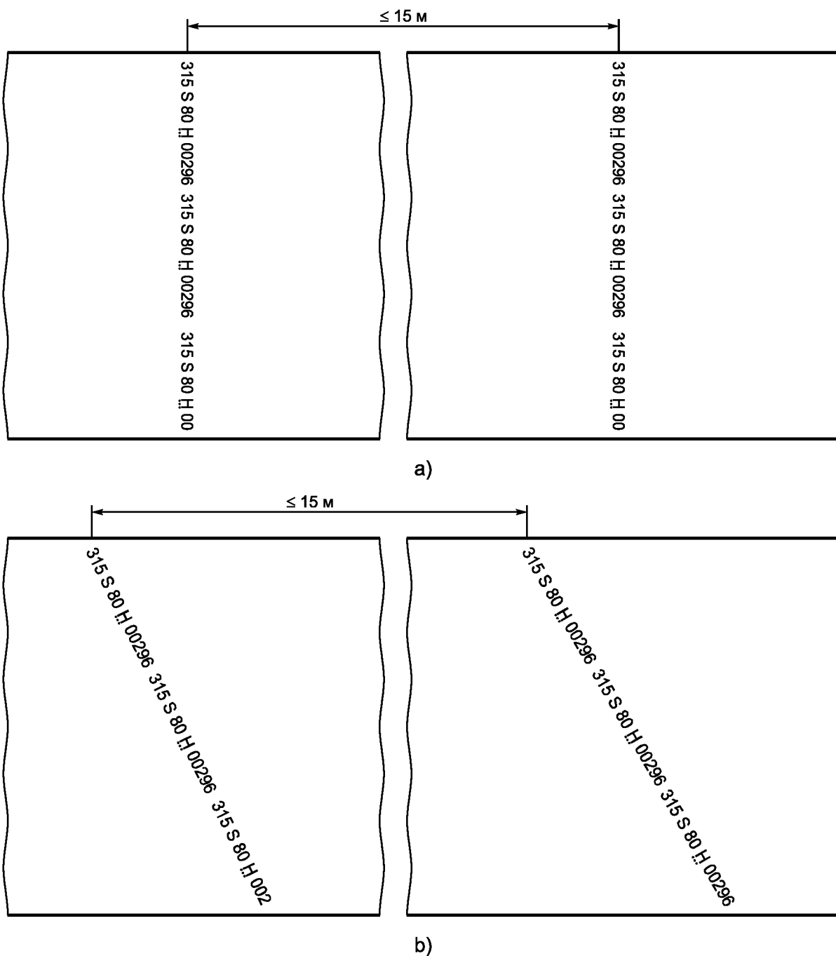
Рисунок 2 — Маркировка полотна ленты
