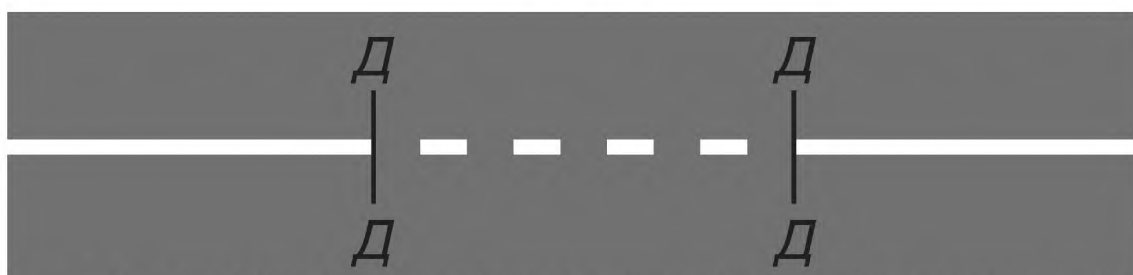
Д-Д – граница сплошной одиночной линии и прерывистой одиночной линии с соотношением штриха к расстоянию между ними 1:1
