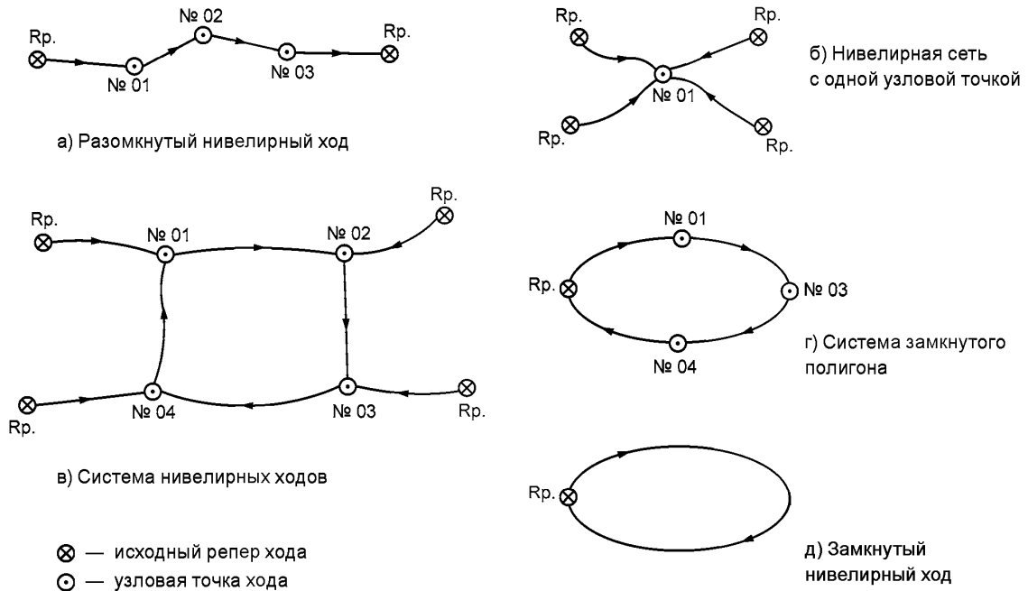
Рисунок 1 — Виды нивелирного хода
