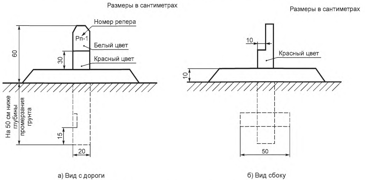
Рисунок Г.1 — Закладка реперов долговременного закрепления
