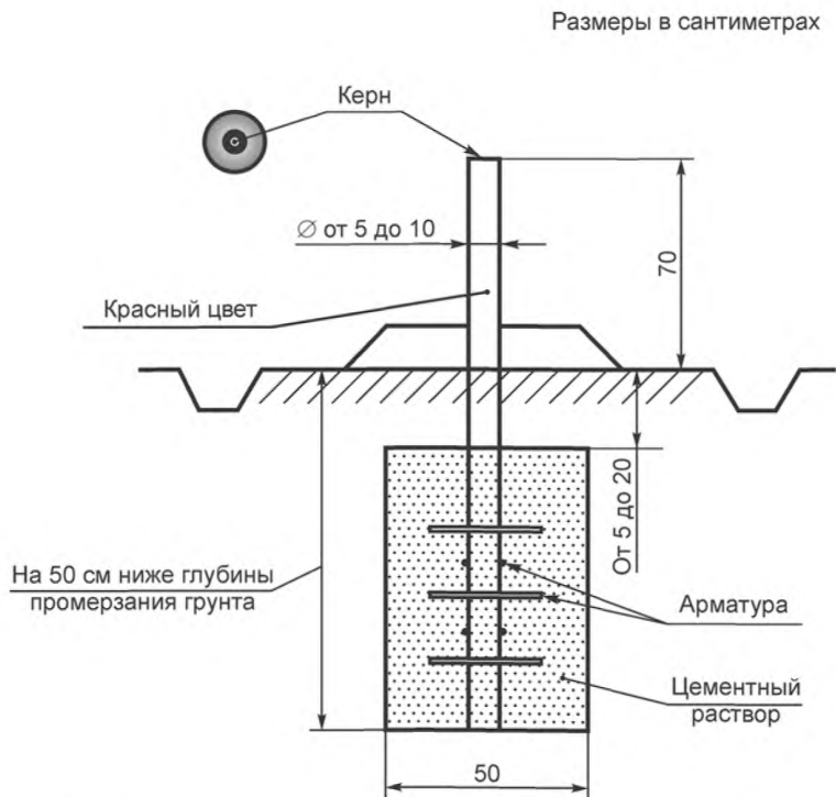
Рисунок Г.2 — Закладка геодезических пунктов долговременного закрепления
