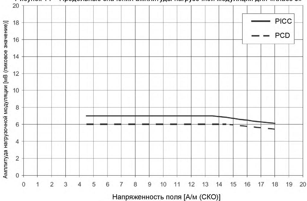
Рисунок 14 – Предельные значения амплитуды нагрузочной модуляции для «Класс 5»
