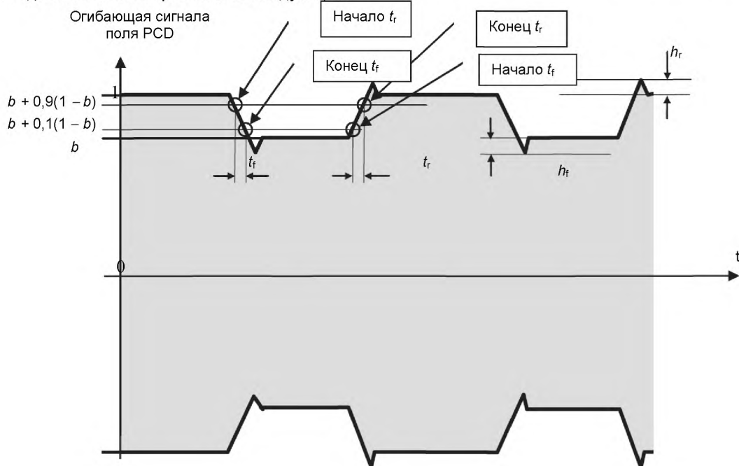
Рисунок 16 – Колебательный сигнал типа В
