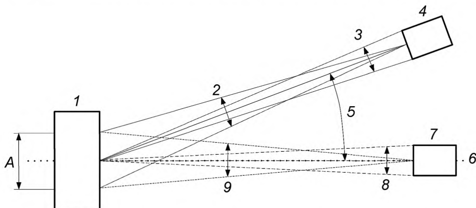
А — диаметр участка тестовой панели; 1 — тестовая панель; 2 — угол не более 3^\circ ; 3 — угол не более 2^\circ ; 4 — искусственный источник света; 5 — угол \beta_B , равный 10^{+0,1^\circ}_{-0,1^\circ} , и угол \beta_B , равный 5^{+0,1^\circ}_{-0,1^\circ} , для L3^* ; 6 — координатная ось; 7 — яркомер; 8 — угол не более 0,5^\circ ; 9 — угол не более 3^\circ
