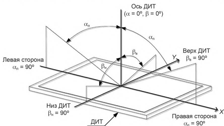
Рисунок 9.1 — Определение углов обзора
