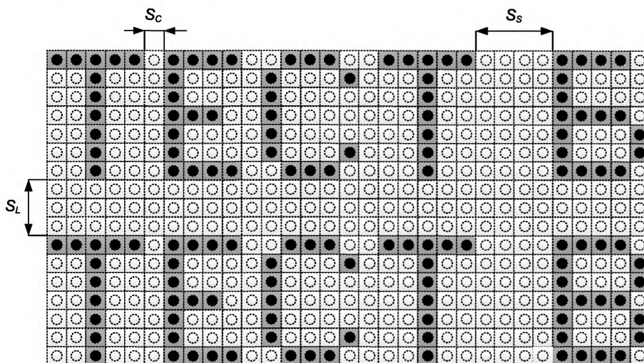
Рисунок 7.1 — Размеры текстовой информации на примере полноматричного экрана
