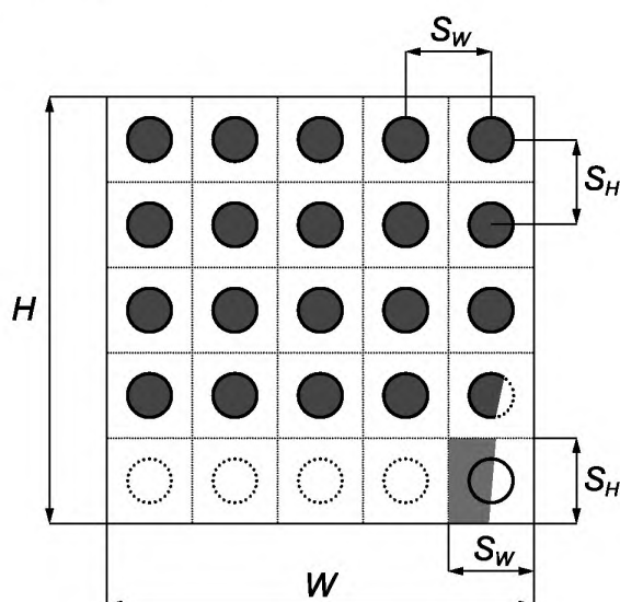
Рисунок 19.2 — Участок тестовой панели из 25 (5·5) элементов
