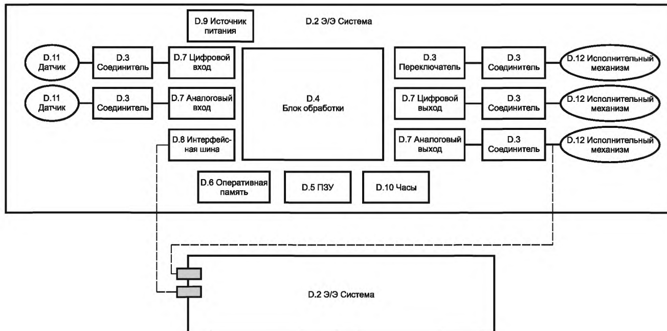
Рисунок D.1 — Общая структура аппаратных средств системы
