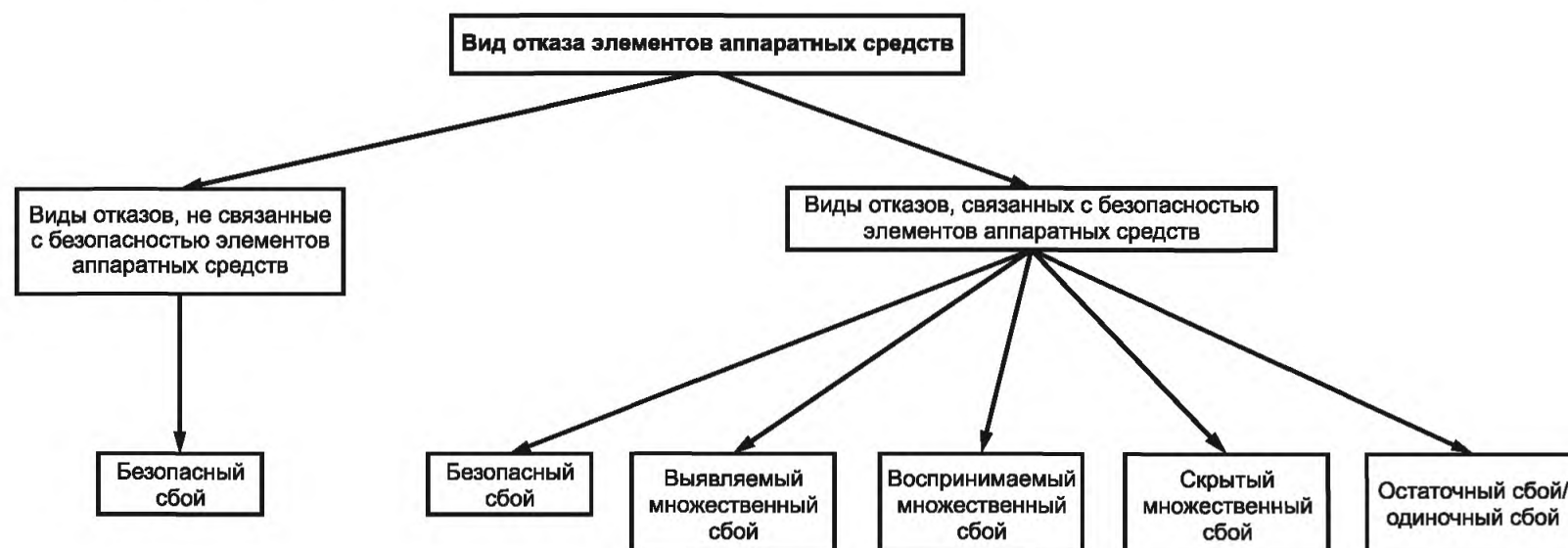
Рисунок В.1 — Классификация видов отказов элементов аппаратных средств
