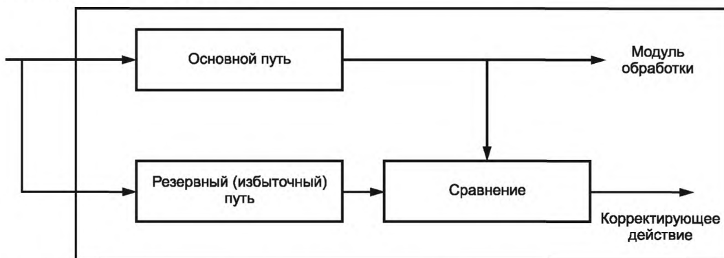
Рисунок D.2 — Сравнение избыточного программного обеспечения в одном модуле обработки
