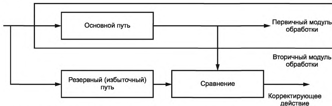
Рисунок D.3 — Сравнение избыточного программного обеспечения на различных модулях обработки
