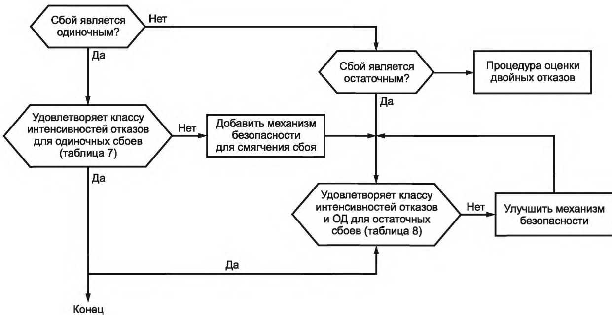
Рисунок 3 — Процедура оценки для одиночных и остаточных сбоев
