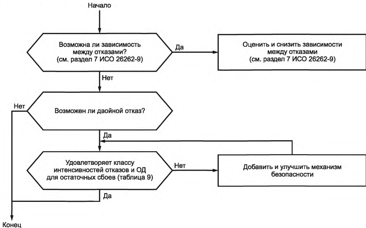
Рисунок 4 — Процедура оценки двойных отказов
