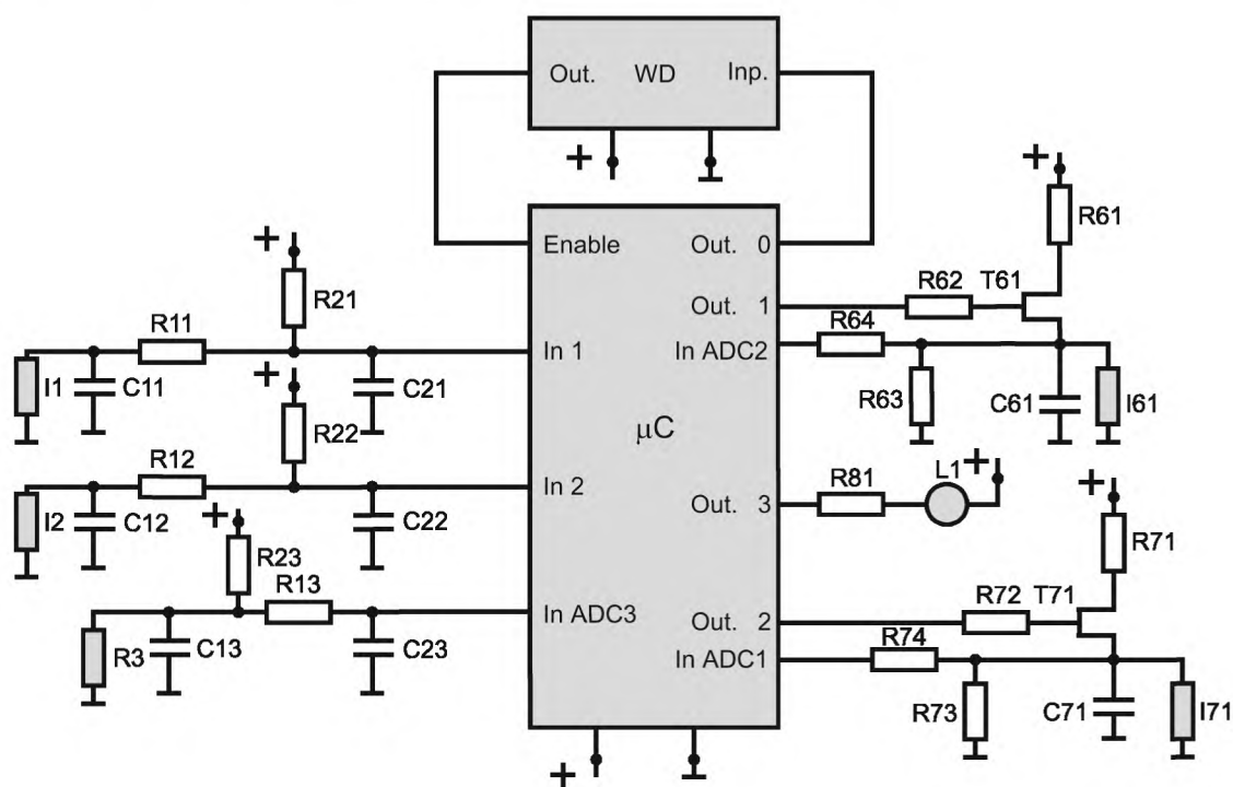
Рисунок Е.1 — Схема рассматриваемого примера
