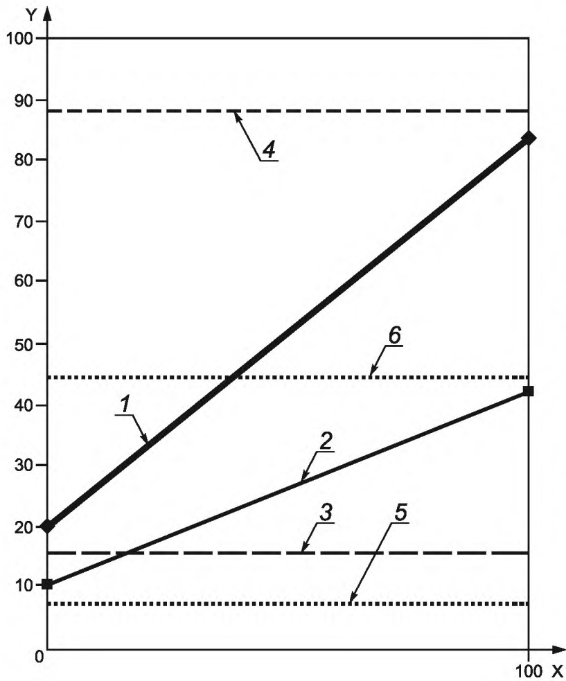
X — физическое показание датчика в %; Y — измеренное показание датчика в % от опорного напряжения; 1 — датчик 1; 2 — датчик 2; 3 — нижняя граница диапазона датчика 1; 4 — верхняя граница диапазона датчика 1; 5 — нижняя граница диапазона датчика 2; 6 — верхняя граница диапазона датчика 2
