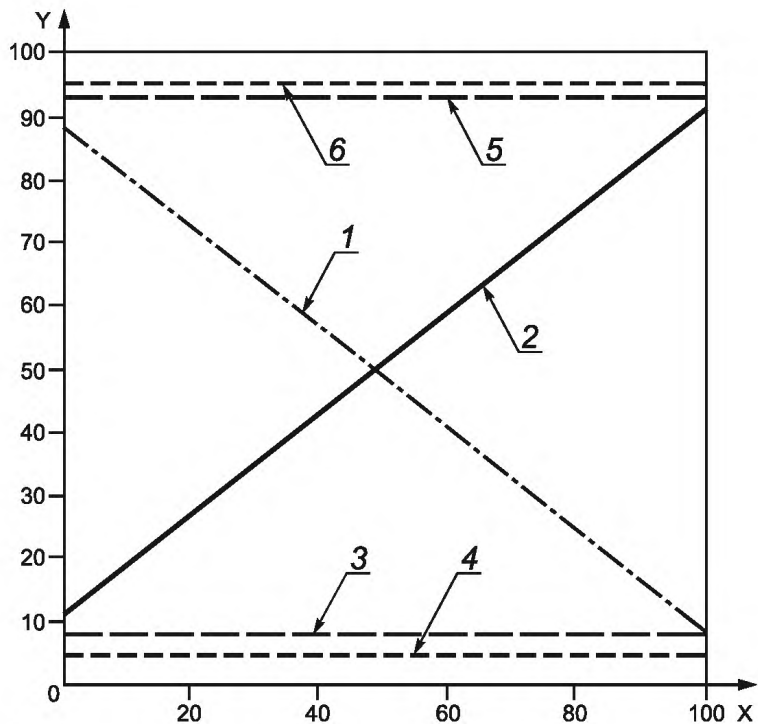
X — физическое показание датчика в %; Y — измеренное показание датчика в % от опорного напряжения; 1 — датчик 1; 2 — датчик 2; 3 — нижняя граница диапазона датчика 1; 4 — нижняя граница диапазона датчика 2; 5 — верхняя граница диапазона датчика 1; 6 — верхняя граница диапазона датчика 2
