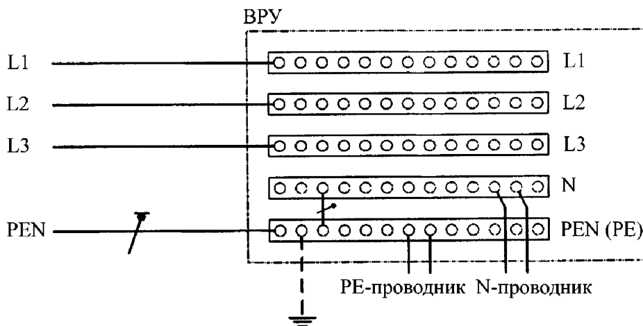
Рисунок А.1 – Подключение PEN-проводника питающей линии к шине PE вводно-распределительного устройства
