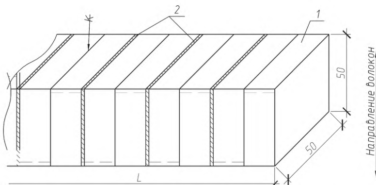
1 – заготовка для образца; 2 – пропили; 3 – припуск на обработку Рисунок 2 – Схема изготовления образцов
