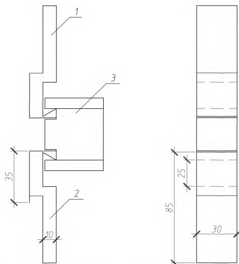
1 – верхняя скоба; 2 – нижняя скоба; 3 – образец
