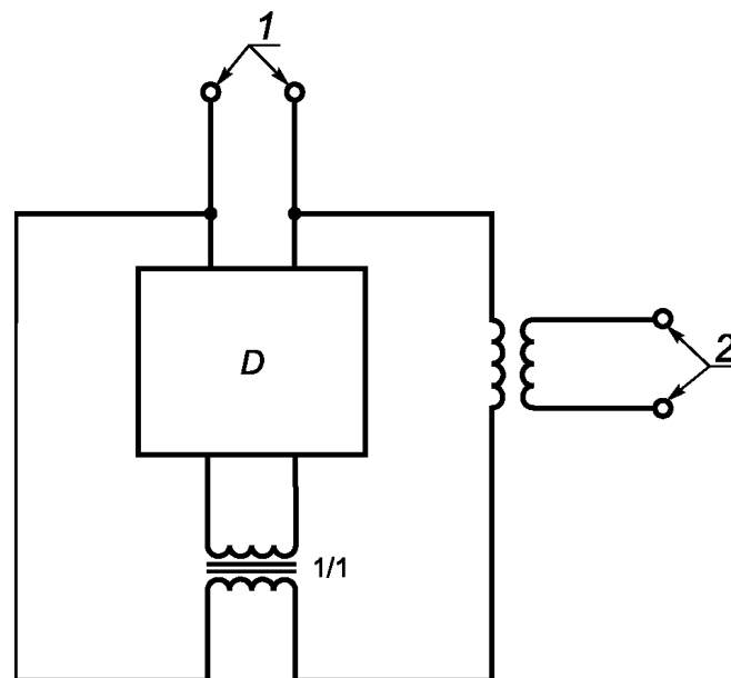
Рисунок 25 — Пример испытательной цепи для проверки старения электронных компонентов (см. 9.23)
