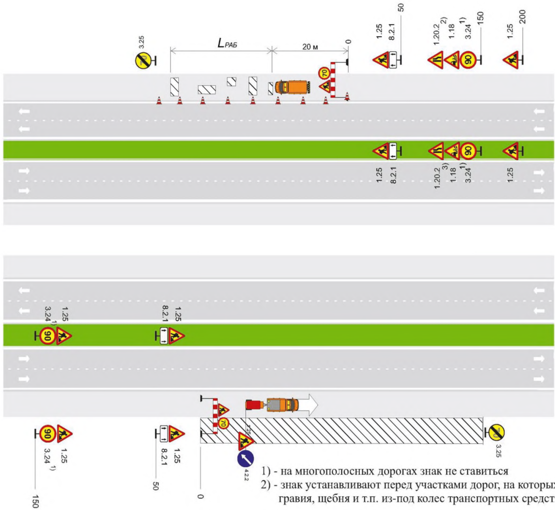
Рисунок Б.37 - Автомагистраль, скоростная дорога, многополосная дорога обычного типа. Рабочая зона краткосрочных работ на обочине или откосе
