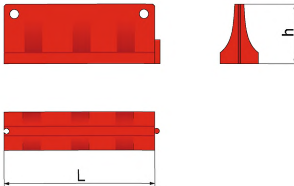
Рисунок 7 – Защитный блок из полимерного материала
