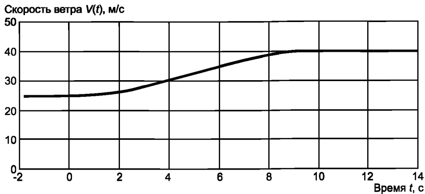
Рисунок 7 — Пример ЭГП ветра ( V_{hub} = 25 м/с)
