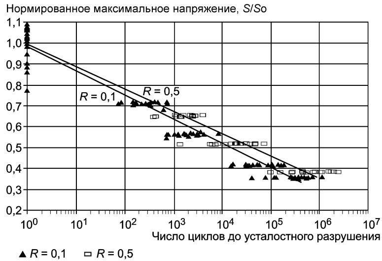
Рисунок Д.2 — Характерные усталостные кривые S - N для композиционного материала на основе стекловолкна
