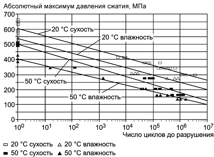
Рисунок Д.3 — Характерные зависимости прочности композиционного материала на основе стекловолкна от влажности
