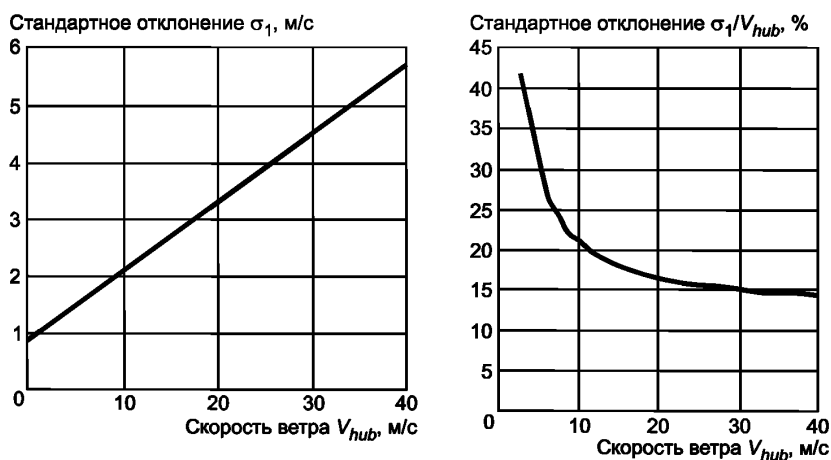
Рисунок 3 — Стандартные отклонения и интенсивность турбулентности в МНТ
