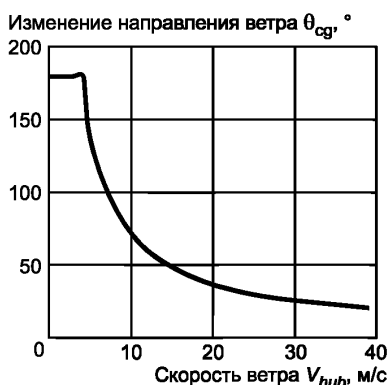
Рисунок 8 — Изменение направления ветра для ЭКН
