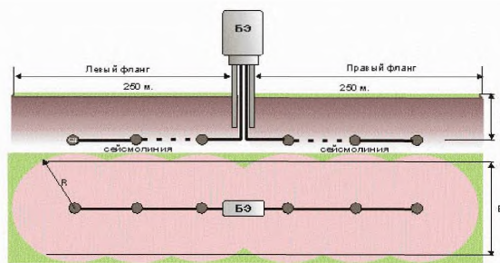
Рисунок 12 – Размещение геофонов
