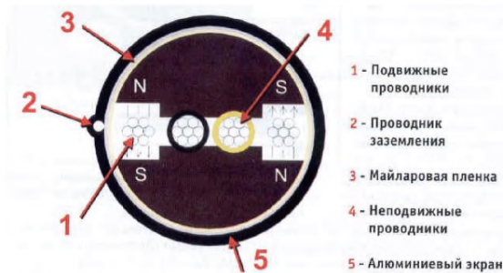
Рисунок 52 - Структура микрофонного кабеля
