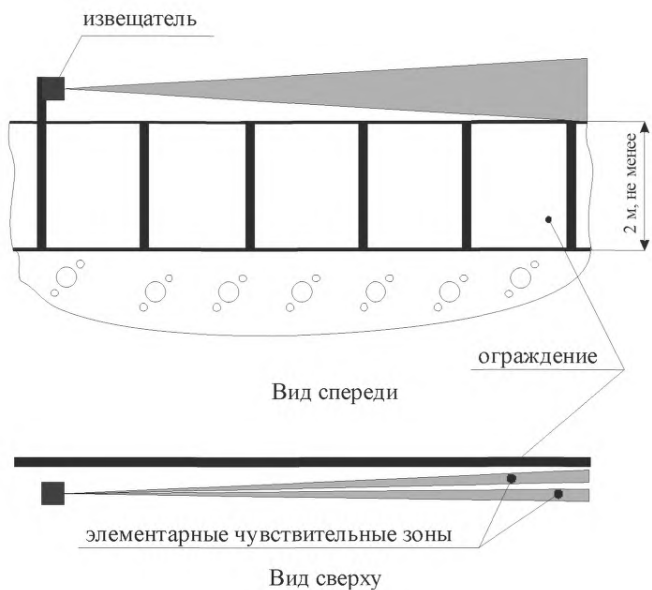
Рисунок 4.16 – Схема блокировки ограждения (забора) «на перелаз»
