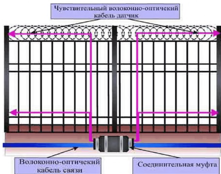
Рисунок 65 – Вариант монтажа системы Ворон™
