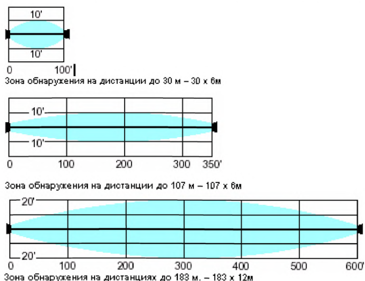
Рисунок 37 – Горизонтальная проекция зоны обнаружения
