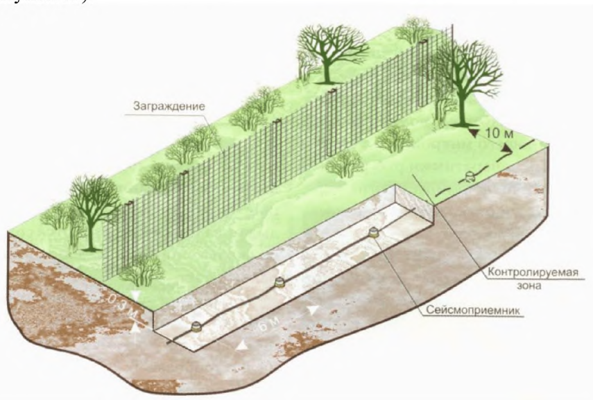
Рисунок 13 – Расположение геофонов среди растительности
