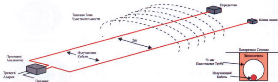
Рисунок 2.78 – ЛВВ – извещатель
