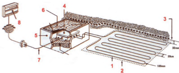
Рисунок 74 - Система SabreLine
