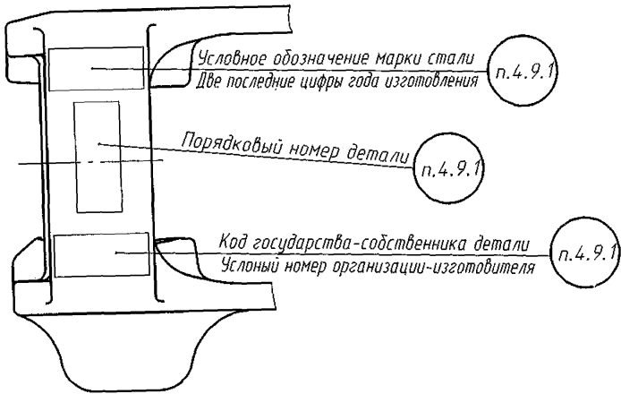
Рисунок И.3 – Расположение знаков маркировки
