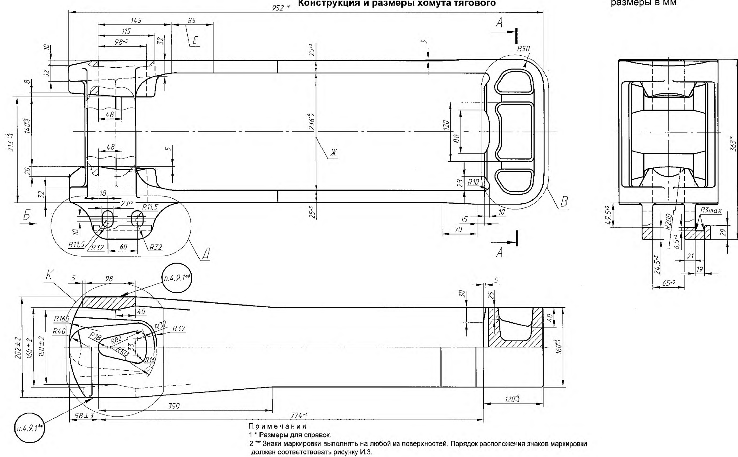
Рисунок И.1 – Хомут тяговый (вариант 1), лист 1
