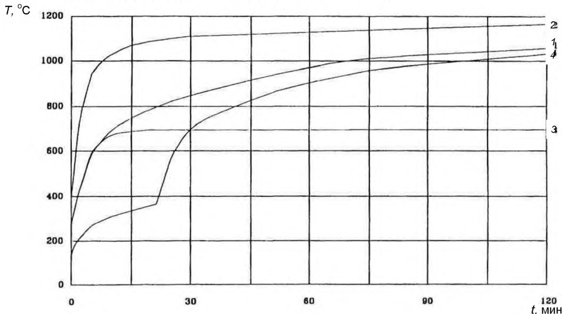
Рисунок 1 – Графики зависимости «температура–время»
