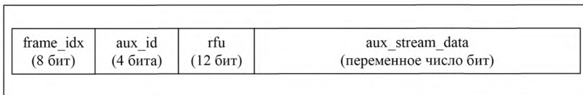
Рисунок 4 — Дополнительный поток как полезная нагрузка
