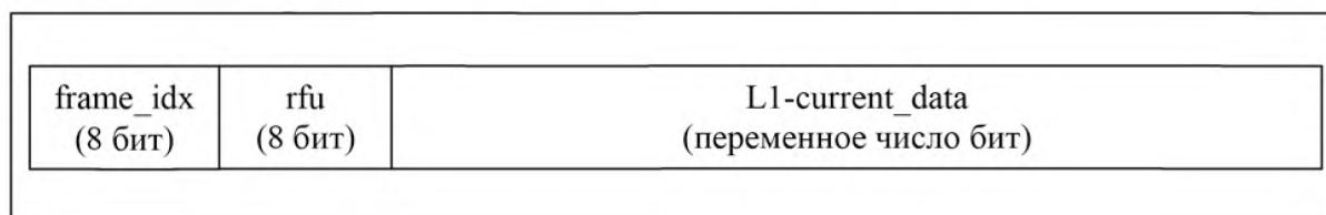
Рисунок 6 — Текущие L1-данные как полезная нагрузка
