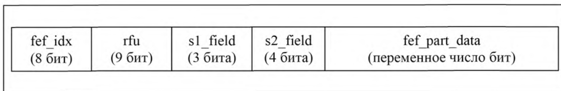
Рисунок 12 — Блок FEF с I/Q-данными как полезная нагрузка
