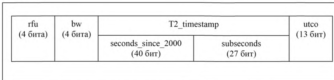
Рисунок 9 — Временной штамп DVB-T2 как полезная нагрузка
