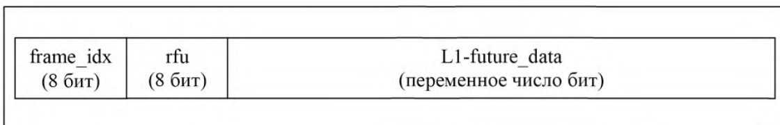
Рисунок 8 — Ячейки балансировки смещения P2 как полезная нагрузка
