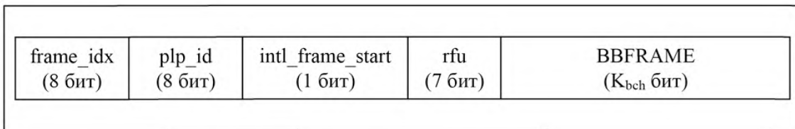
Рисунок 3 — Базовый кадр как полезная нагрузка
