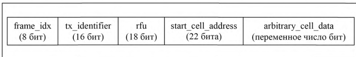
Рисунок 5 — Произвольные ячейки как полезная нагрузка
