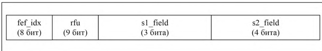
Рисунок 11 — Нулевой блок FEF как полезная нагрузка
