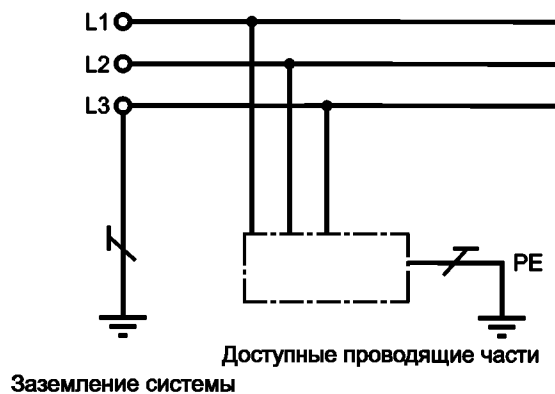
Рисунок Б.4 — ТТ система
