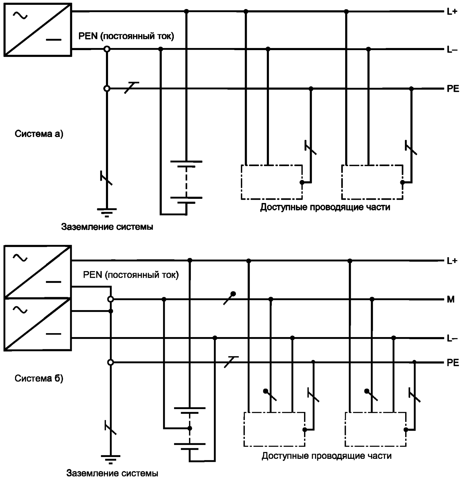
Рисунок Б.5 — TN-S система постоянного тока
