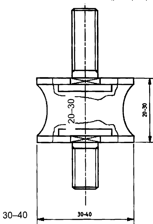
Рисунок 4 — Типичная резиновая втулка для крепления испытательной панели
