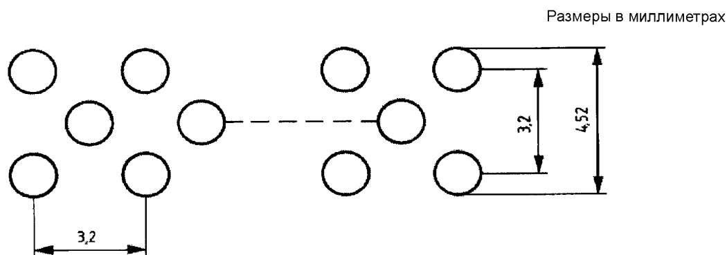
Рисунок 5 — Фронтальная поверхность рабочей части горелки
