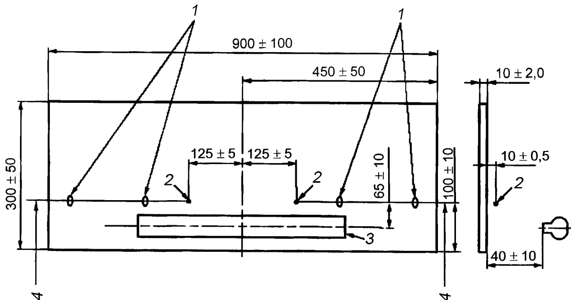
Рисунок А.1 — Расположение системы измерения температуры
