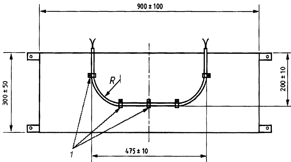
Рисунок 7 — Способ крепления образца при испытании
