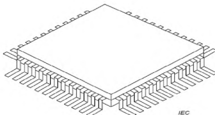
Рисунок 9 – корпус типа PLQFP (квадратный)
