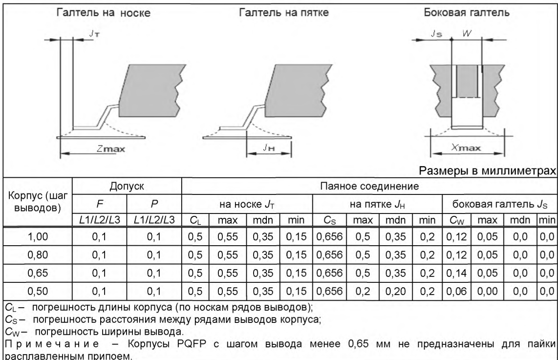
Рисунок 7 – Анализ формы паяного соединения
