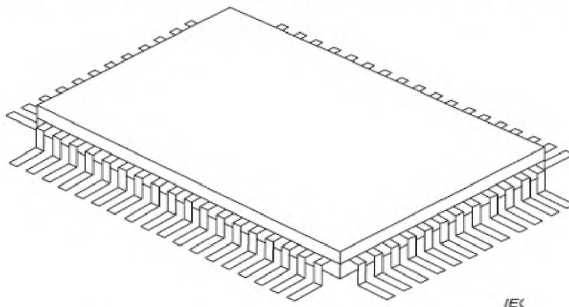
Рисунок 5 – Конструкция корпуса типа PQFP (прямоугольный)
