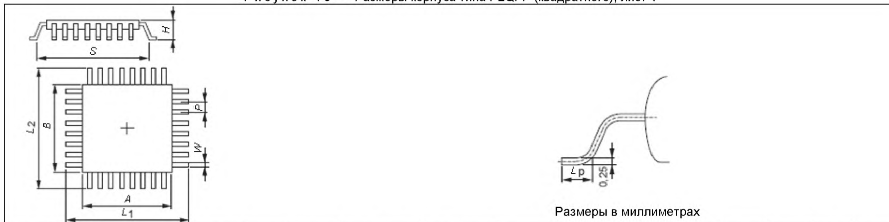
Рисунок 10 – Размеры корпуса типа PLQFP (квадратного), лист 1
