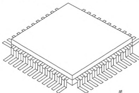
Рисунок 1 – Конструкция корпуса типа PQFP (квадратный)
