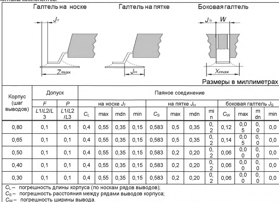
Рисунок 19 – Анализ формы паяного соединения
