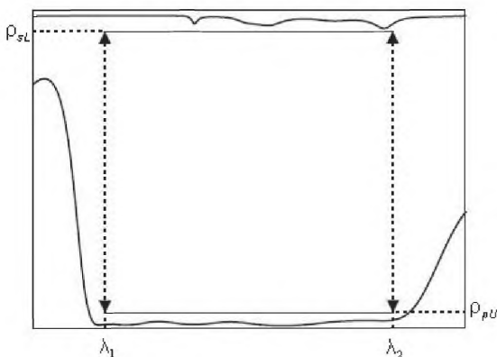
Рисунок 9 – Поляризующая функция
