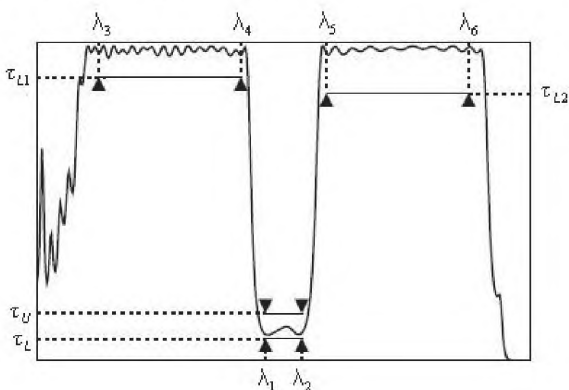
Рисунок 6 – Заграждающая функция
