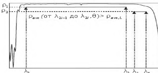
Рисунок 1 – Отражающая функция
