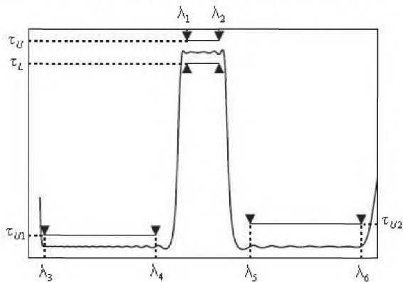
Рисунок 5 – Пропускающая функция
