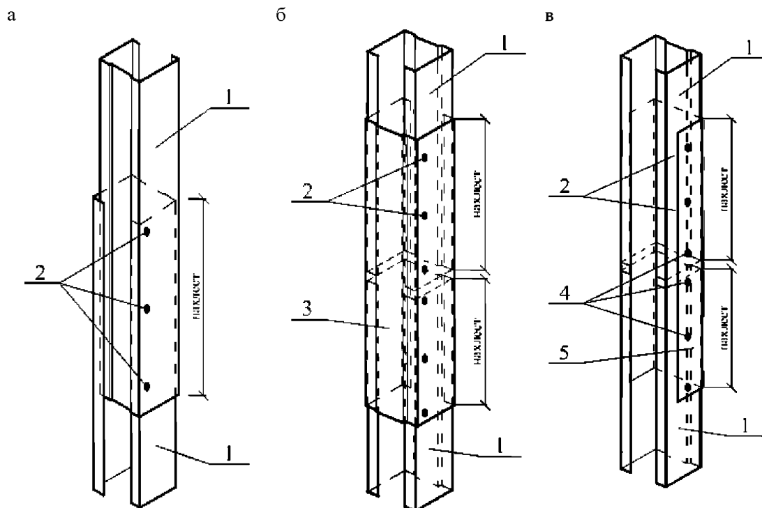
а – 2 ПС-профиля соединены в виде коробки; б – 2 ПС-профиля соединены встык и объединены в виде коробки дополнительным ПС-профилем; в – 2 ПС-профиля соединены встык и объединены дополнительным ПН-профилем 1 – ПС-профиль; 2 – самонарезающий винт; 3 – добавочный ПС-профиль; 4 – просечка; 5 – добавочный ПН-профиль
