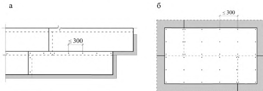
Рисунок Е.5.4 – Схема закрепления пола винтами
