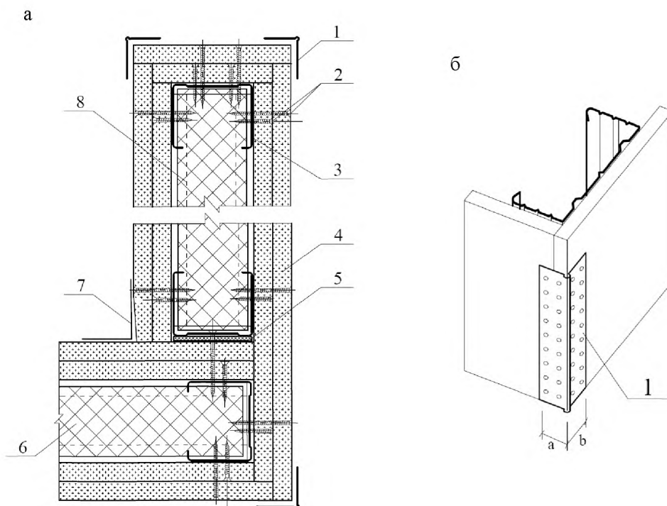
а – угол перегородки из гипсокартонных или гипсоволокнистых листов; б – схема установки ПУ-профиля на наружный угол перегородки 1 – ПУ-профиль; 2 – самонарезающий винт; 3 – ПС-профиль; 4 – лист ГКЛ или ГВЛ; 5 – лента уплотнительная; 6 – тепло- звукоизоляционный материал; 7 – армирующая лента с заполнением шва; 8 – ПН-профиль
