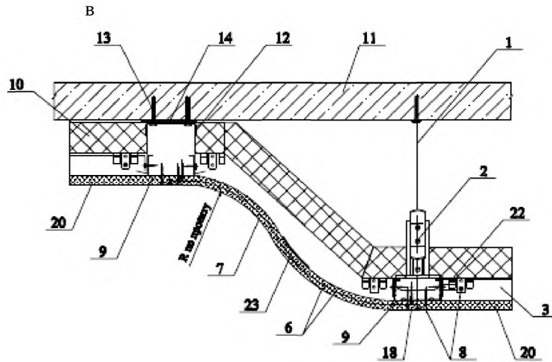
а – пример вогнутого цилиндрического свода, выполненного гнутыми профилями; б – пример облицовки потолочной балки (радиус кривизны от 100 до 400 мм); в – пример выполнения разноуровневого потолка
