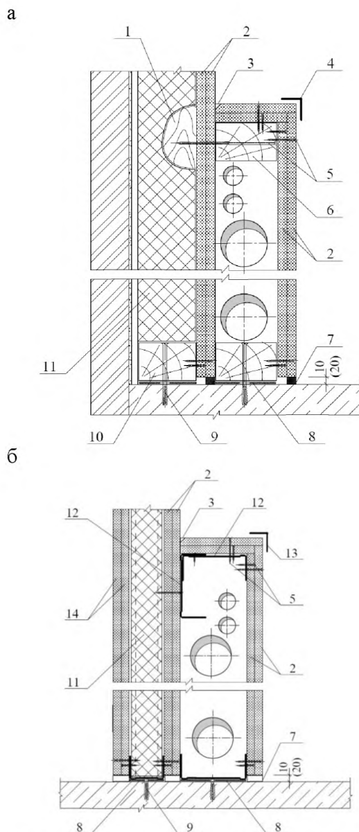
а – размещенных вдоль капитальной стены; б – вдоль перегородки 1 – стоечный брус; 2 – лист ГКЛ или ГВЛ влагостойкий; 3 – шпаклевка; 4 – PL-профиль; 5 – самонарезающий винт; 6 – брус; 7 – герметик; 8 – уплотнительная лента; 9 – дюбель-гвоздь; 10 – брус; 11 – тепло- звукоизоляционный материал
