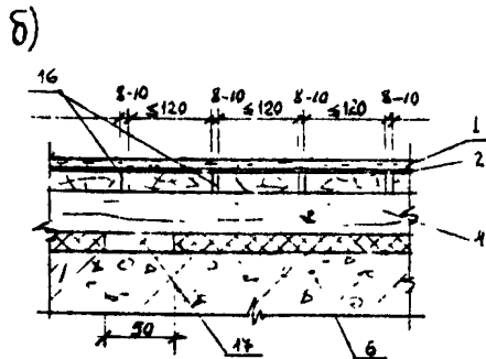
Рис. 2 КОНСТРУКТИВНЫЕ МЕРЫ ПО ОСУЩЕСТВЛЕНИЮ ПОДПОЛЬНОГО ПРОСТРАНСТВА
