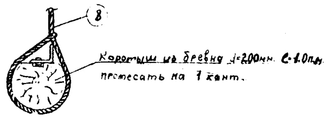
Рис. 12 Узел строповки опоры П220 337 КРЯК КРОНА К-162
