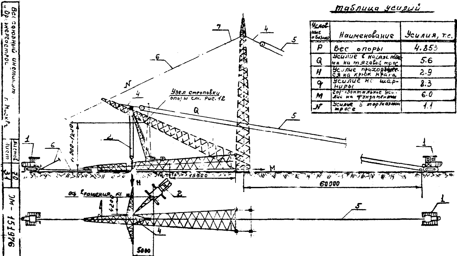
Рис. 10 Схема подъема опоры ПЭД-3 краном К-162 и 2 ми тракторами.
