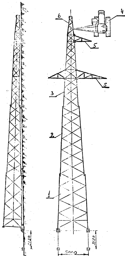
Рис.14 Пристыковка траверсы и тросостойки к стволу опоры
