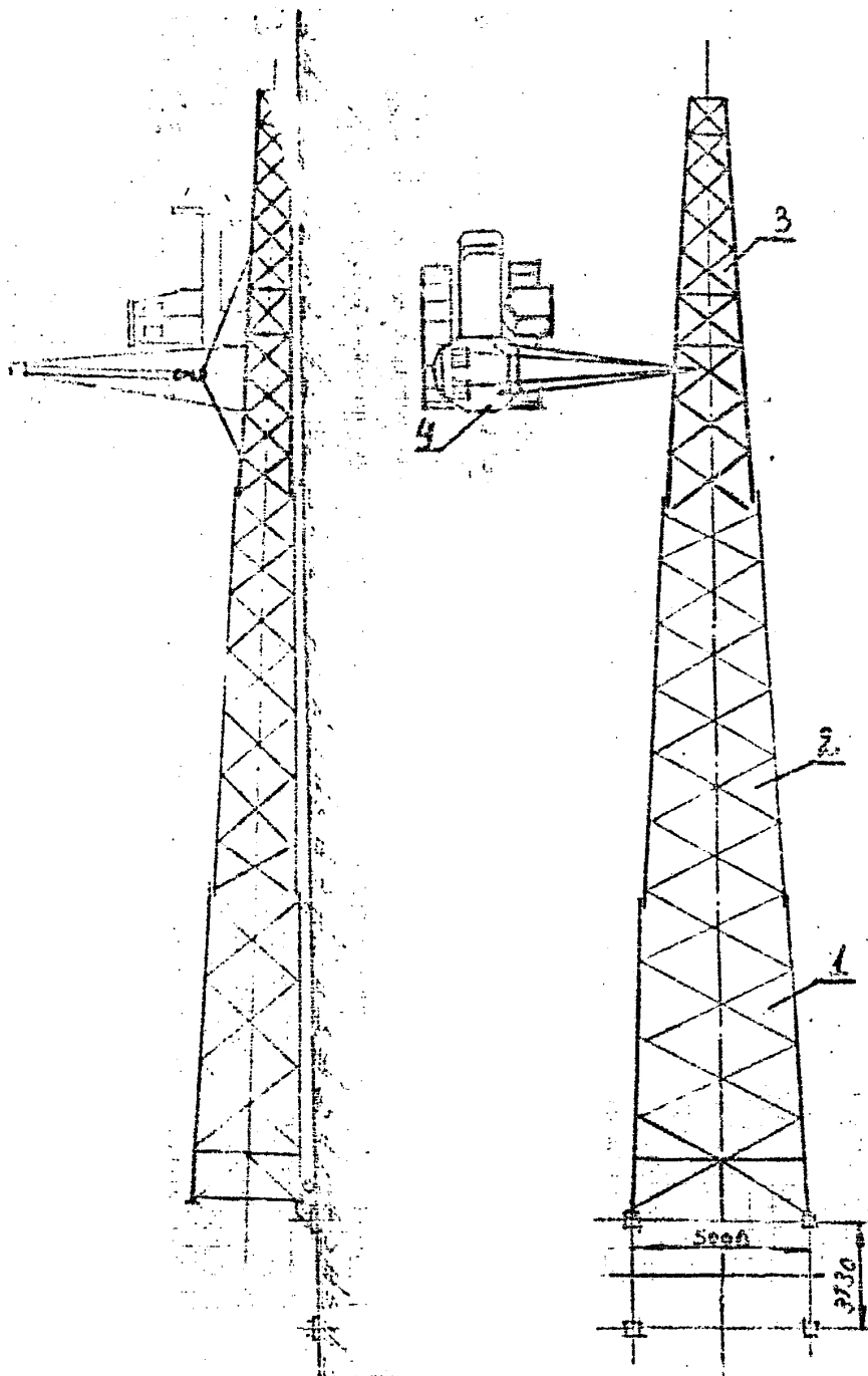
Рис. 13 Пристыковка 3 ей секции ствола опоры П220-3
