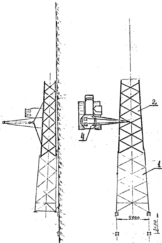
Рис. 12 Пристыковка 2 ой секции ствола опоры 17220-3
