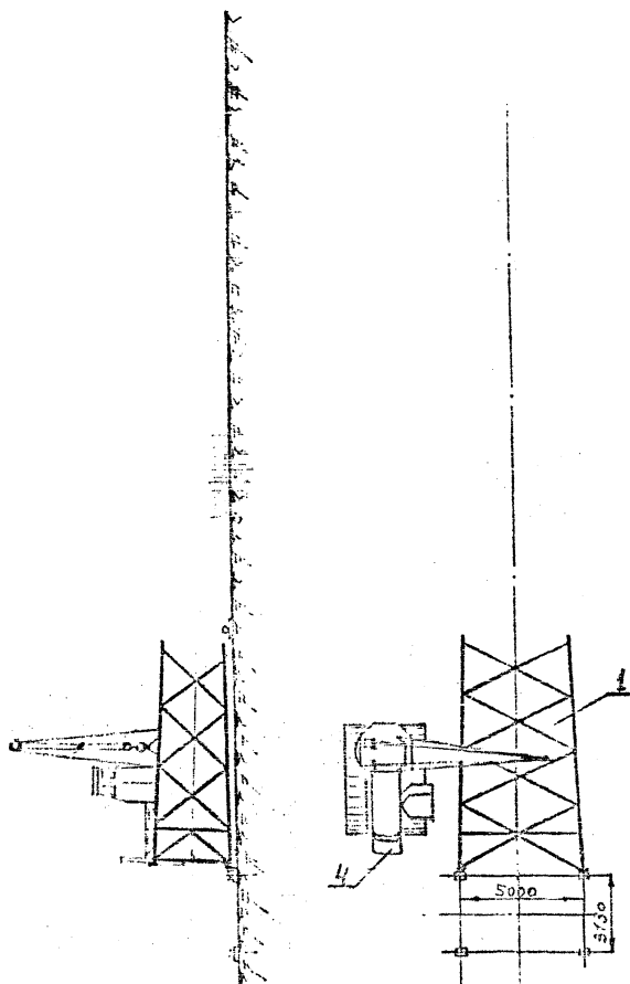
Рис. II Сборка 100 ой секции ствола опоры П220-3
