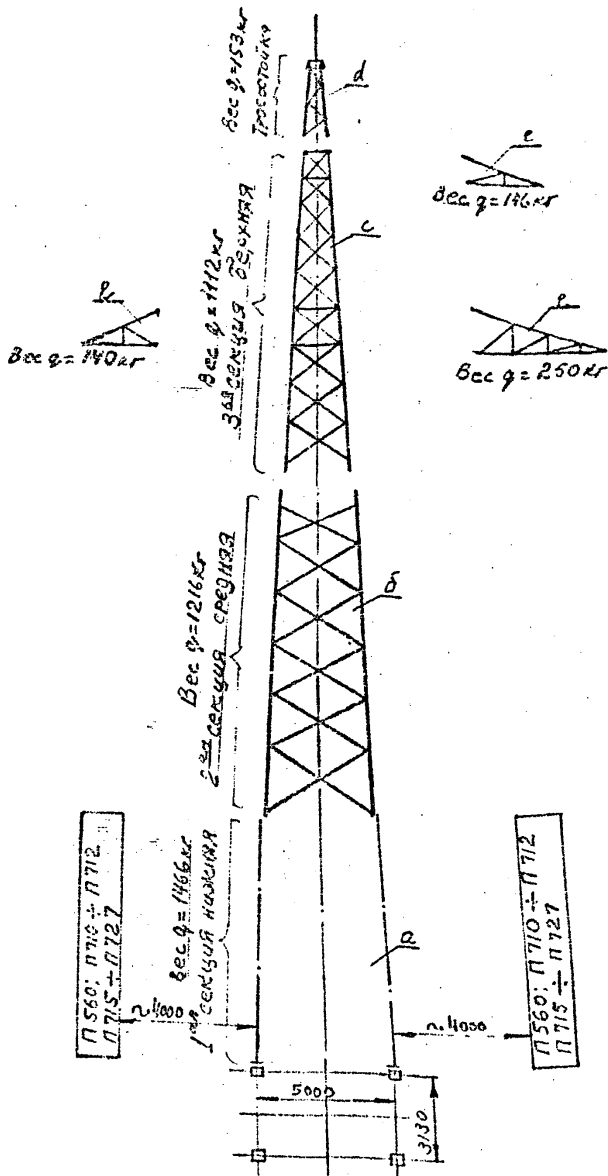
Рис. 10 Раскладка пакетов и секций опоры П 220-3 на высоте
