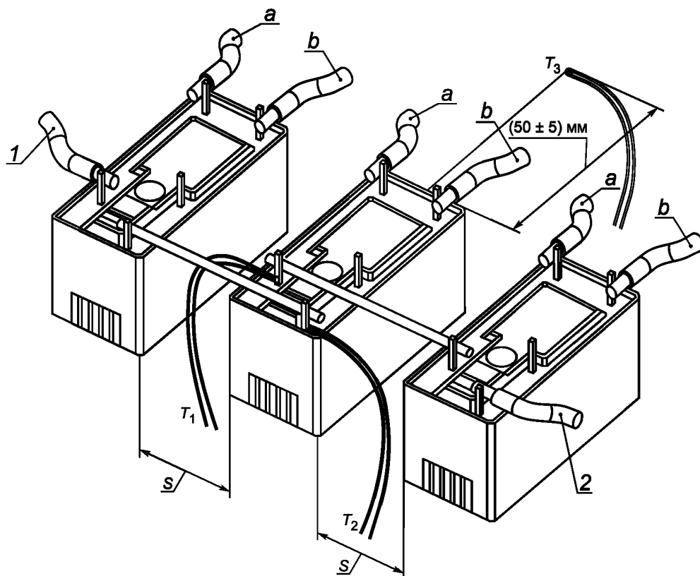
1, 2 — клеммы контактов; a, b — клеммы катушки; S — установочное расстояние; T_1 — термопары.
