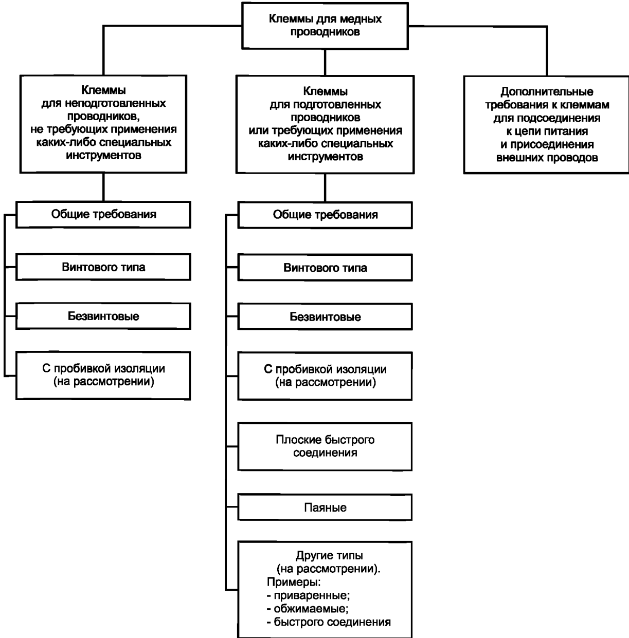
Рисунок J.1 — Схема семейств клемм
