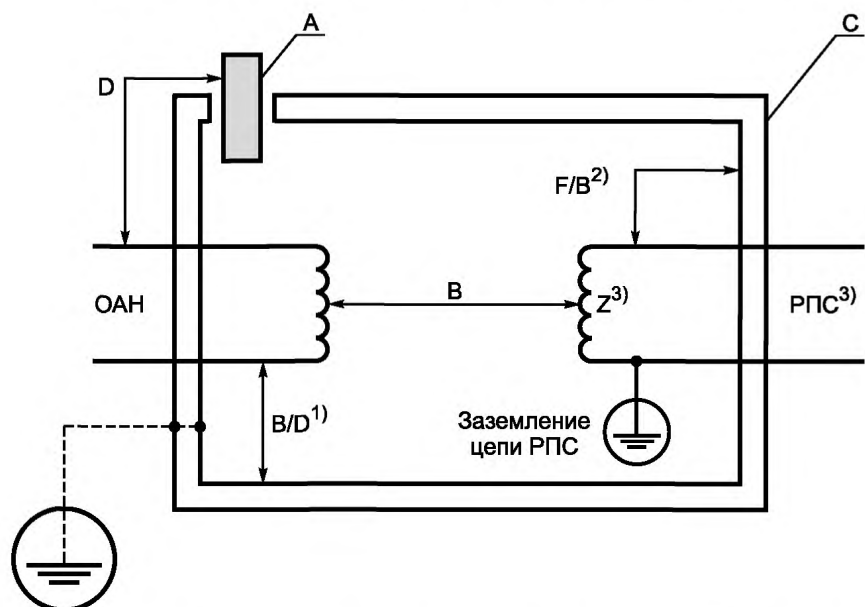
Рисунок А.2 — Оборудование с входом/выходом (I/O) ЗСНН
