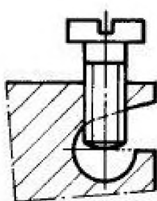
б) винтовой зажим с непосредственным давлением
