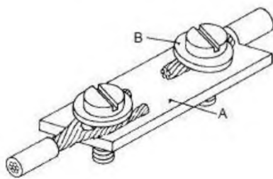
б) пример винтового зажима с передачей давления головкой винта через промежуточную деталь
