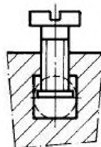
с) с прижимной пластиной
