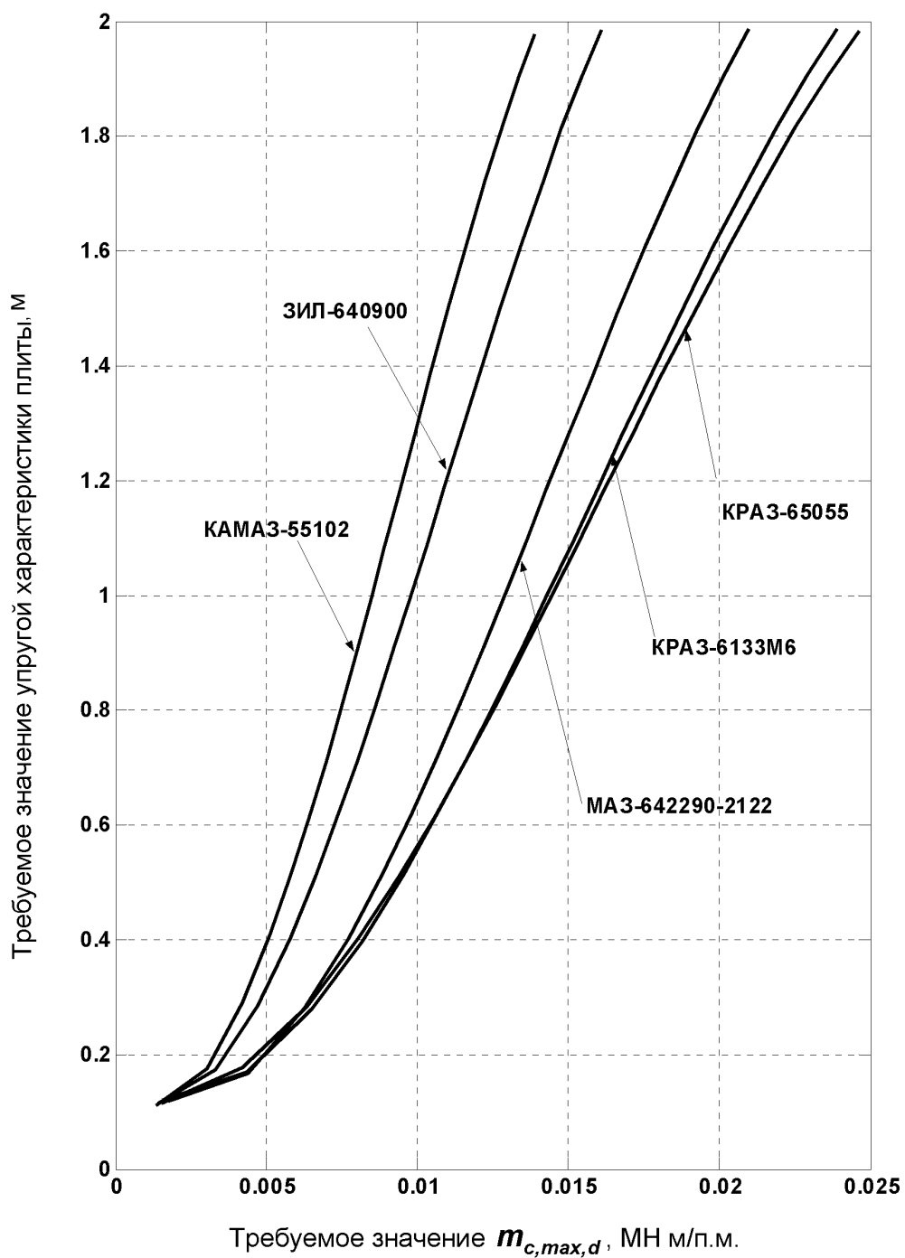
Рисунок 15 - Номограмма для определения I_d для автомобилей
