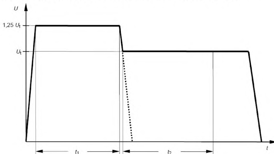
Рисунок 1 – Испытательное напряжение
