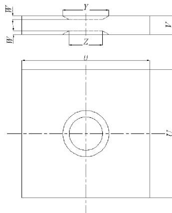
Рисунок Л.3 – Опорная плита
