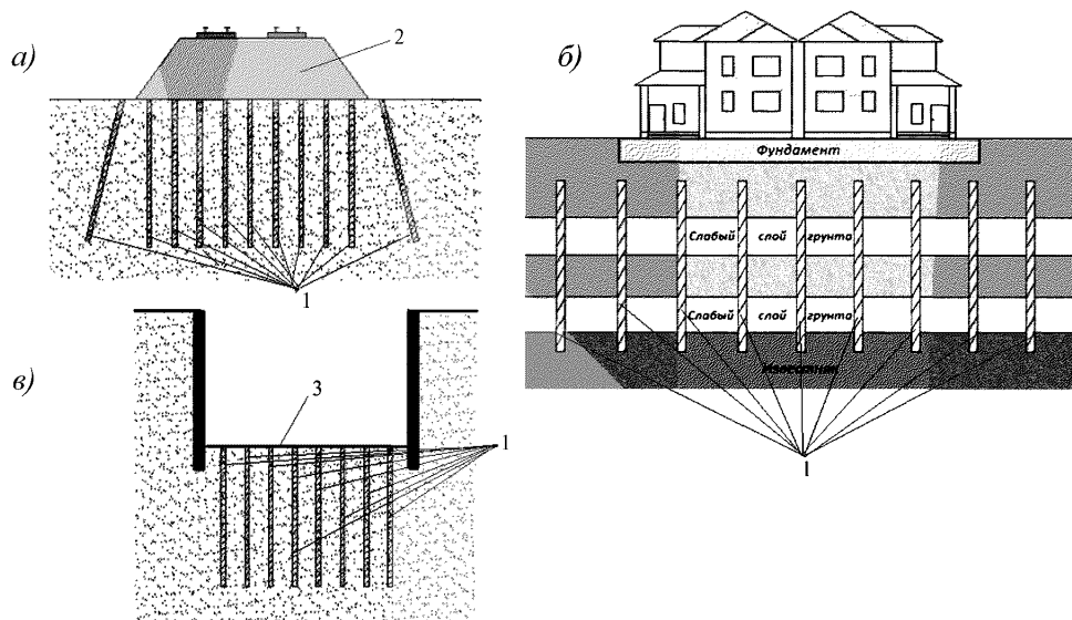
Рисунок 5.5 – Варианты применения микросвай для усиления существующих фундаментов
