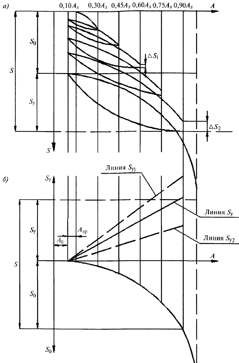
а) – график «усилия-перемещения»; б) – график упругих и остаточных перемещений; A_0 – начальная нагрузка; A_{тр} – потери усилия на трение при преднапряжении; A_s – усилие, соответствующее пределу текучести; S_y – упругие перемещения; S_0 – остаточные перемещения; \Delta S – прирост перемещения; S_{y1} ; S_{y2} – граничные значения перемещений
