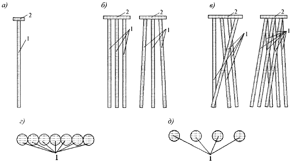
a) – одиночная микросвая; б) – группа (куст) микросвай; в) – сетка из микросвай; з) – стена из микросвай касательного расположения; д) – стена из микросвай прерывистого расположения;
