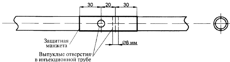
Рисунок 10.4 – Схема расположения выпускных отверстий в инъекционной трубке
