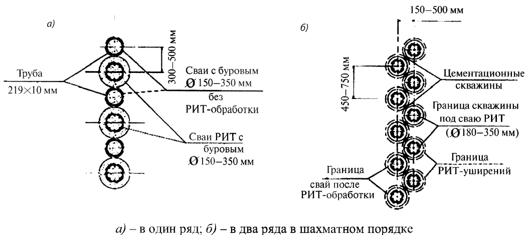
а) – в один ряд; б) – в два ряда в шахматном порядке Рисунок 7.11 – Варианты расположения микросвай РИТ в подпорной стенке*
