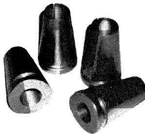
Рисунок 11.10 – Натяжение и закрепление тяги анкера из арматурных канатов при помощи инвентарной обоймы и отдельных запрессовочных конусов
