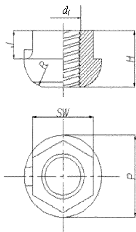
Рисунок Л.1 – Фиксирующая шаровая гайка. Тип 1
