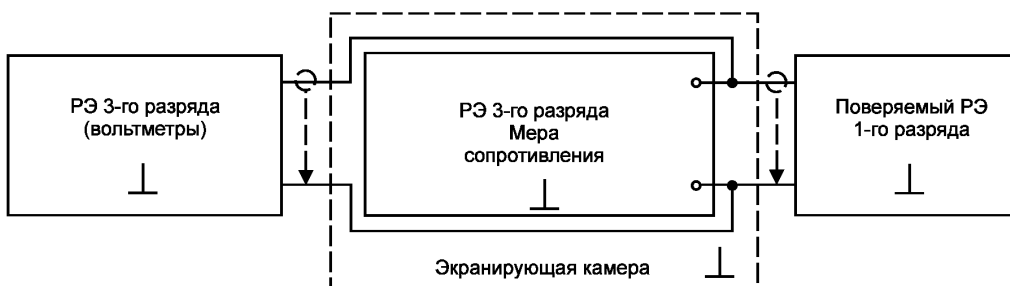
Рисунок 8 — Схема соединения приборов при проверке РЭ 1-го разряда [калибраторы (меры) тока и поверочные установки, работающие в режиме воспроизведения силы тока] в диапазоне от 1 \cdot 10^{-10} до 1 \cdot 10^{-9} А с помощью РЭ, заимствованных из других поверочных схем
