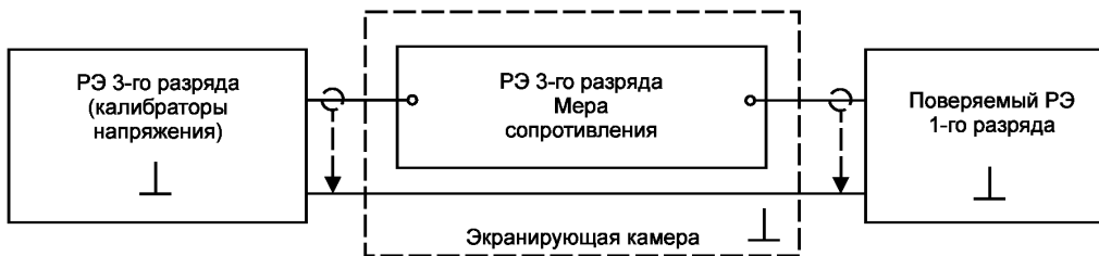
Рисунок 7 — Схема соединения приборов при проверке РЭ 1-го разряда [измерители тока (амперметры) и поверочные установки, работающие в режиме измерения силы тока] в диапазоне от 1 \cdot 10^{-10} до 1 \cdot 10^{-9} А с помощью РЭ, заимствованных из других поверочных схем
