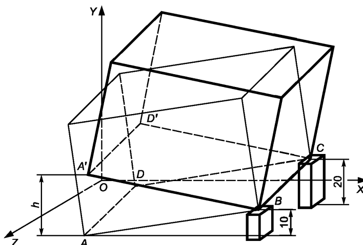
Рисунок 5 — Испытание падением на угол изделия
