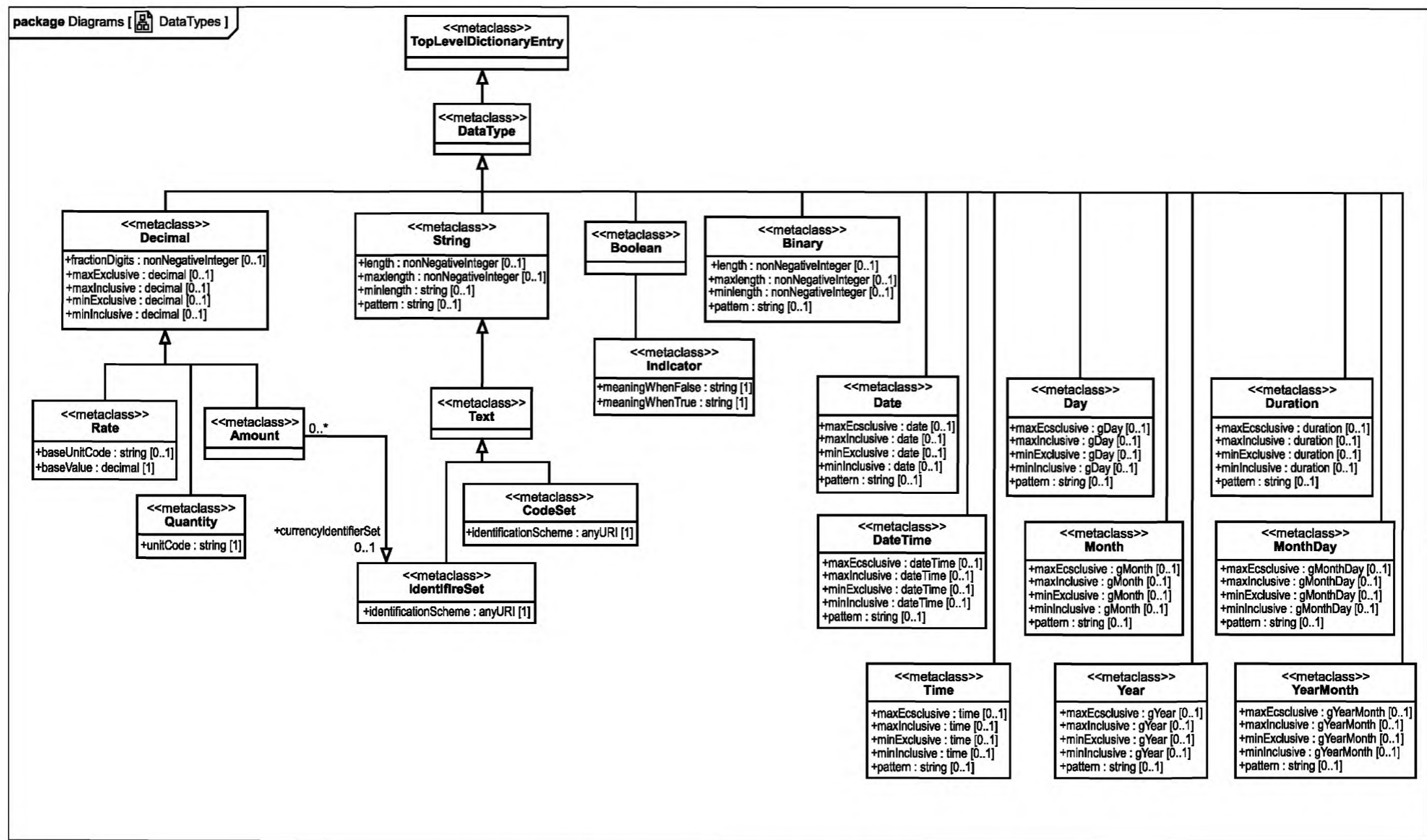
Рисунок 15 — ТипыДанных, определяемые пользователем
