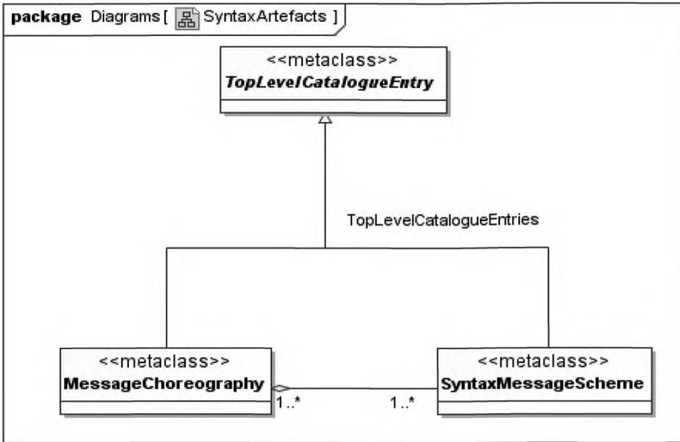
Рисунок 8 — Синтаксис артефактов
