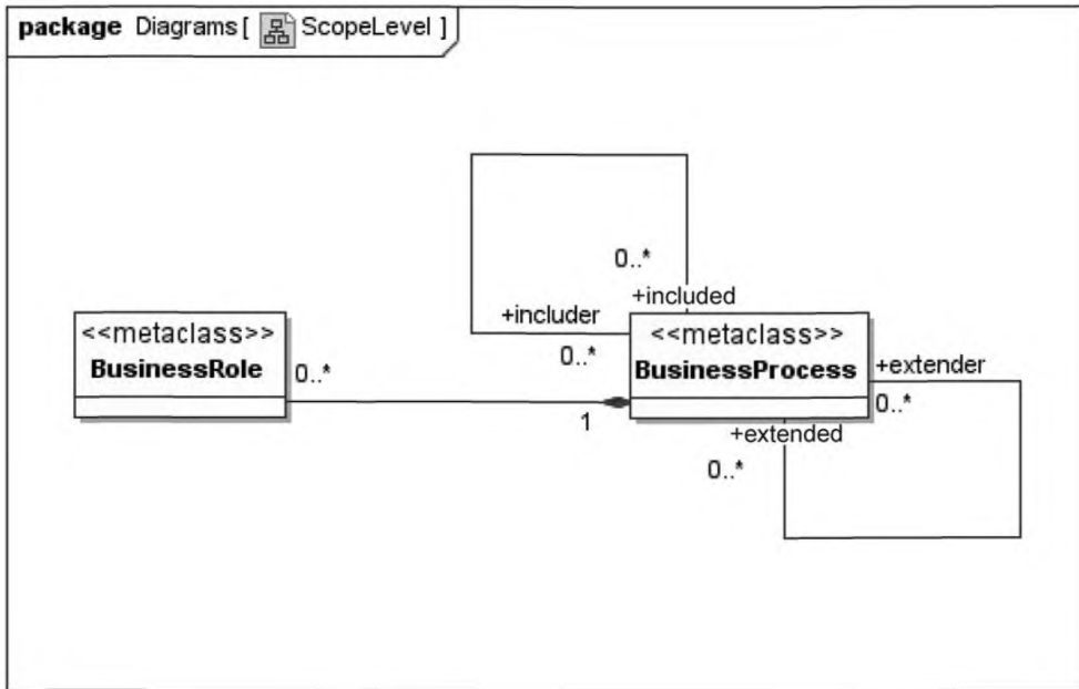
Рисунок 4 — Обзорный уровень
