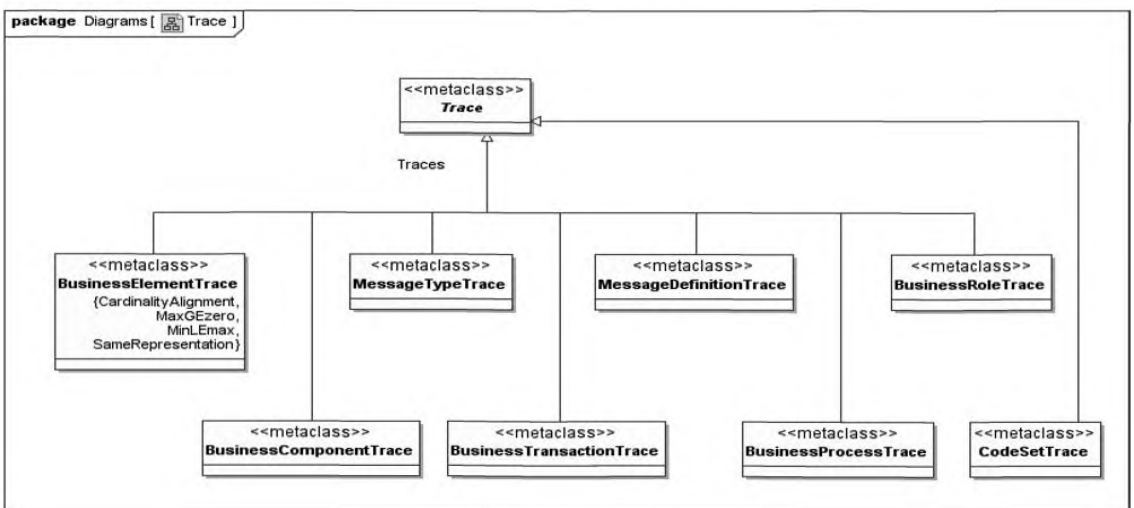
Рисунок 9 — Следы
