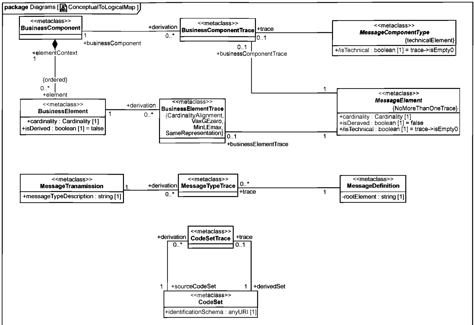
Рисунок 11 — Отображение Концептуального уровня в Логический уровень
