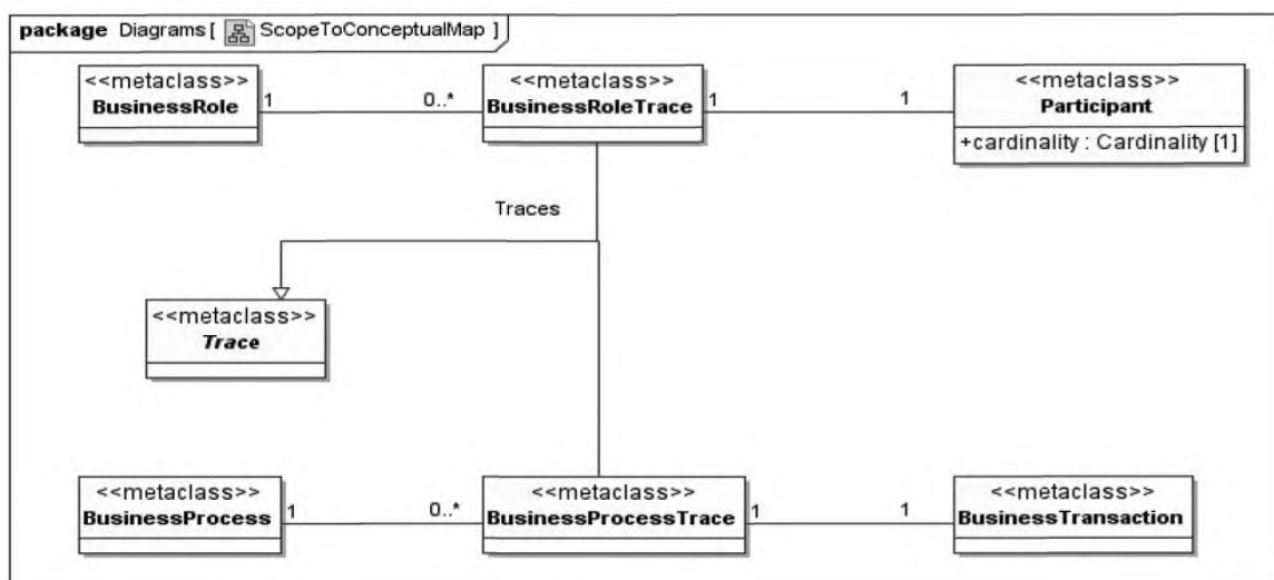
Рисунок 10 — Отображение Обзорного уровня в Концептуальный уровень
