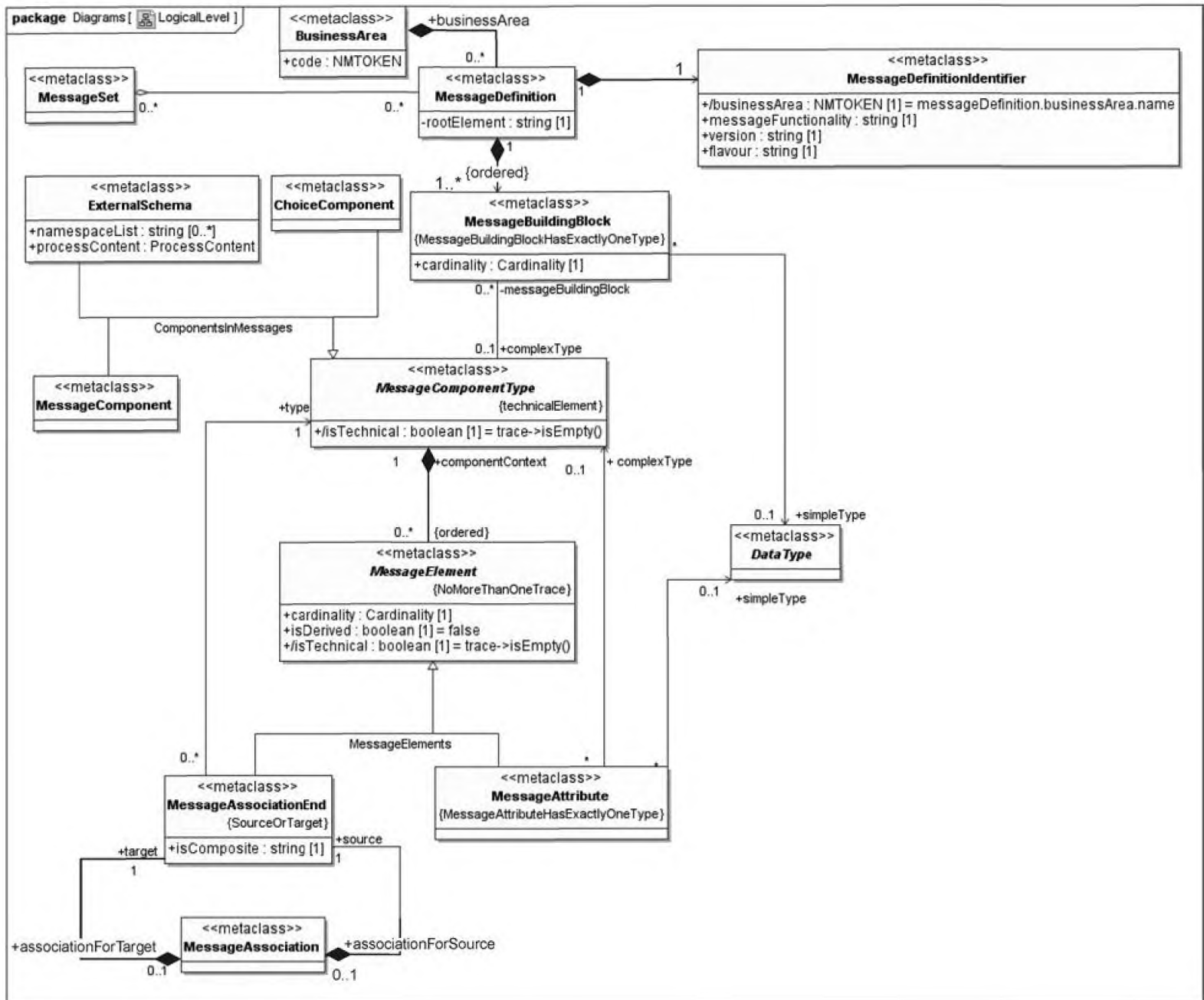
Рисунок 7 — Логический уровень
