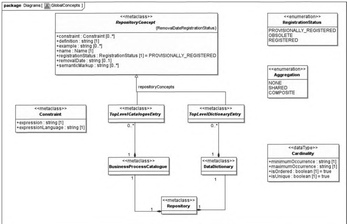
Рисунок 13 — Глобальные концепты
