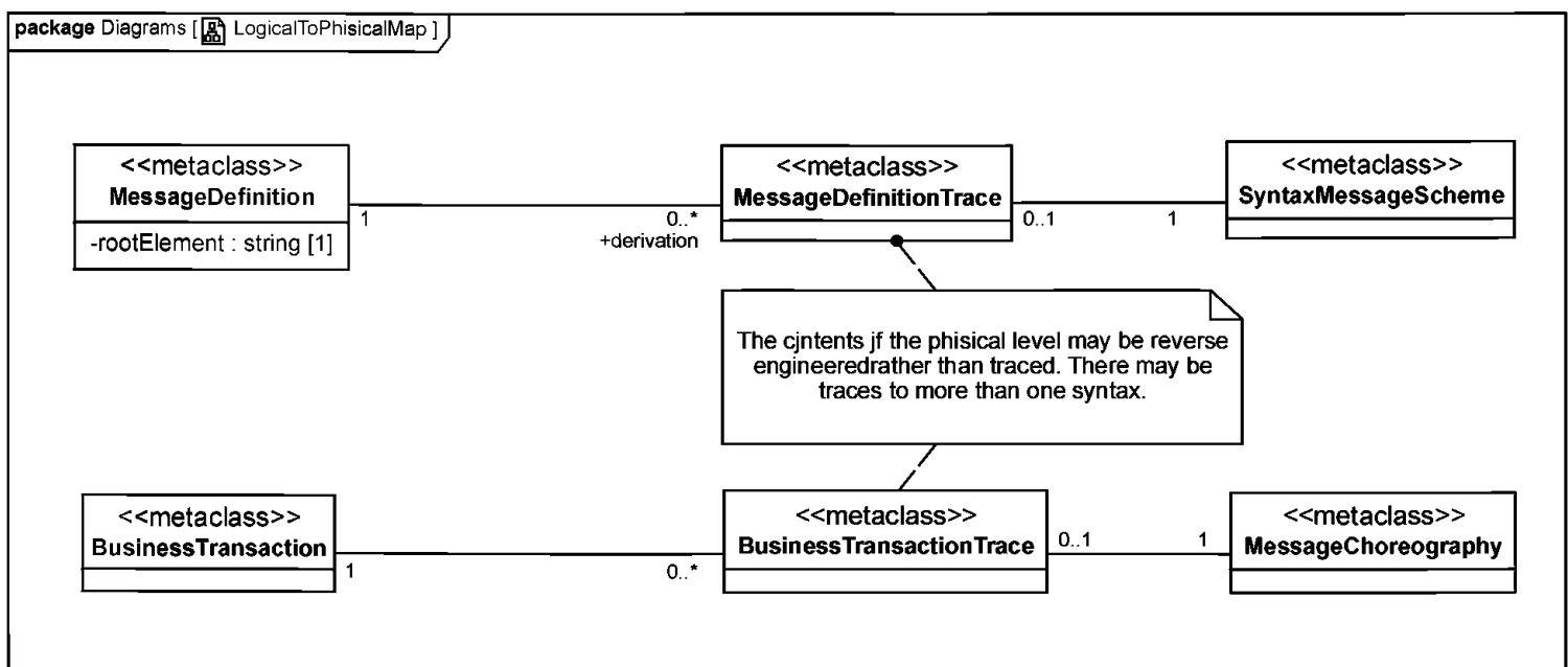
Рисунок 12 — Отображение Логического уровня в Физический уровень
