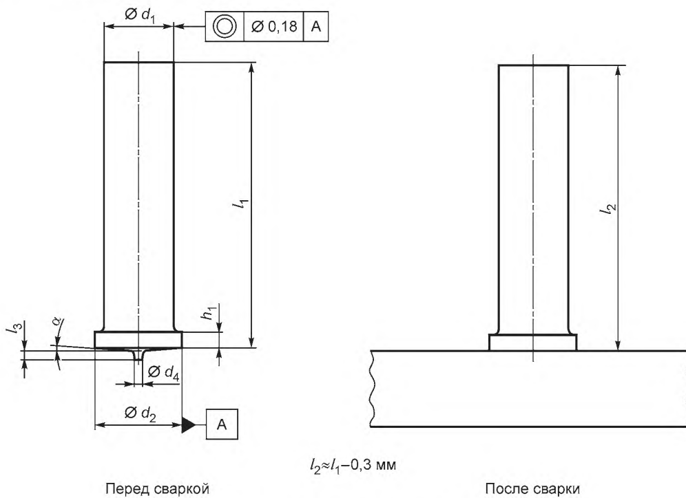
Рисунок 10 — Шпилька без резьбы (UT)
