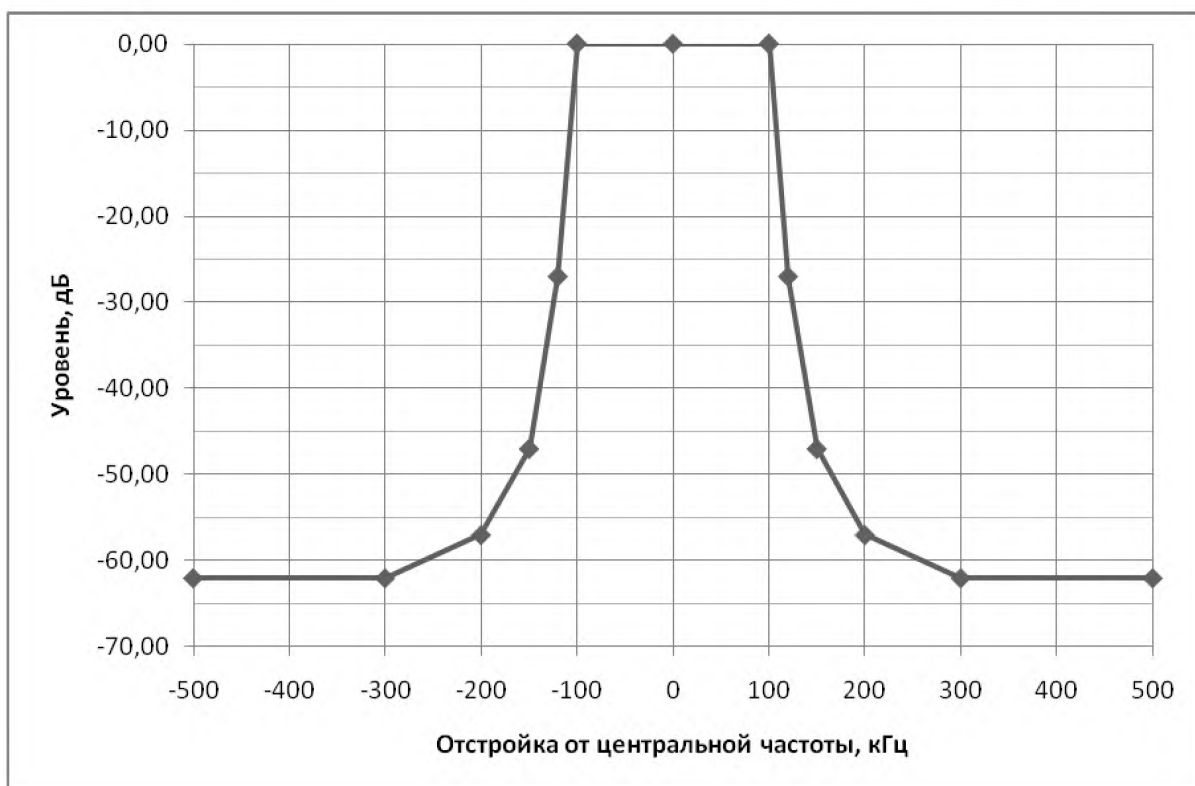
Рисунок 1 – Маска огибающей внеполосных радиокосебаний для ширины полосы частот 100 кГц
