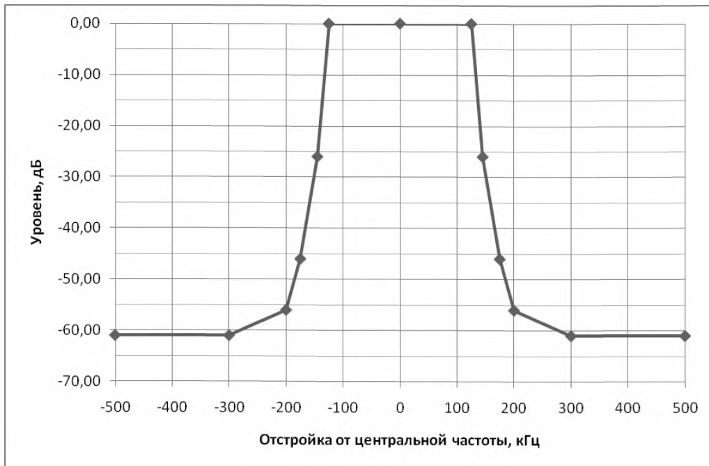
Рисунок 3 – Маска огибающей внеполосных радиополебов для ширины полосы частот 250 кГц
