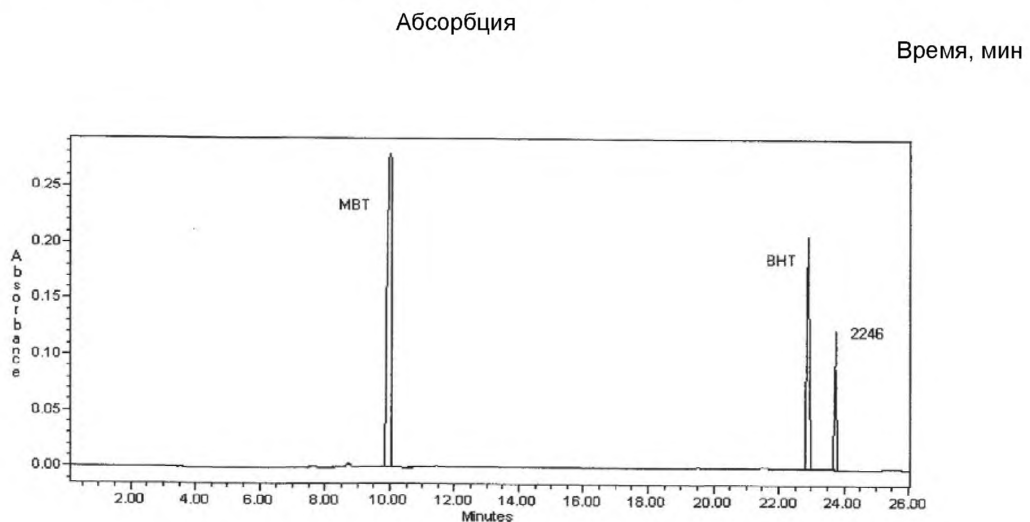
Рисунок А.1 – Хроматограммы для МВТ и антиоксидантов
