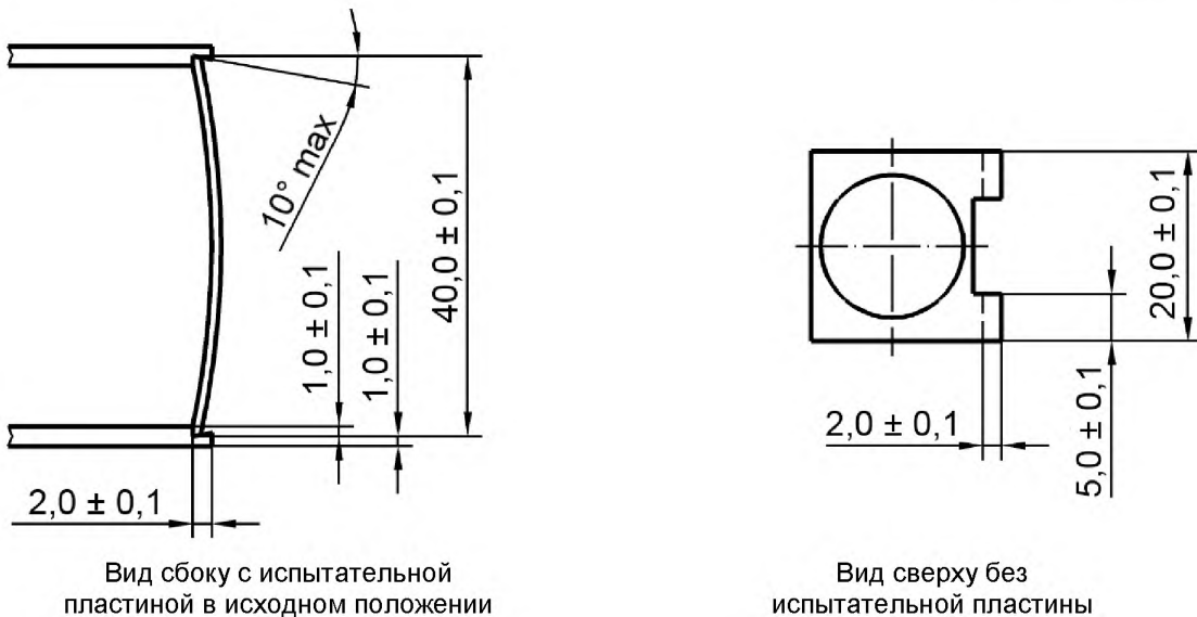
Рисунок 5 – Зажимы
