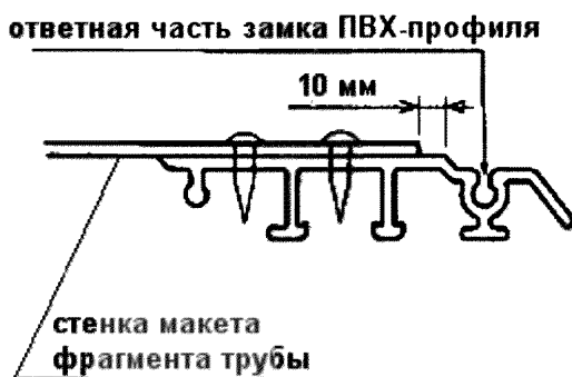
Рисунок 6 – Фиксация кольца из ПВХ-профиля в макете фрагмента трубы
