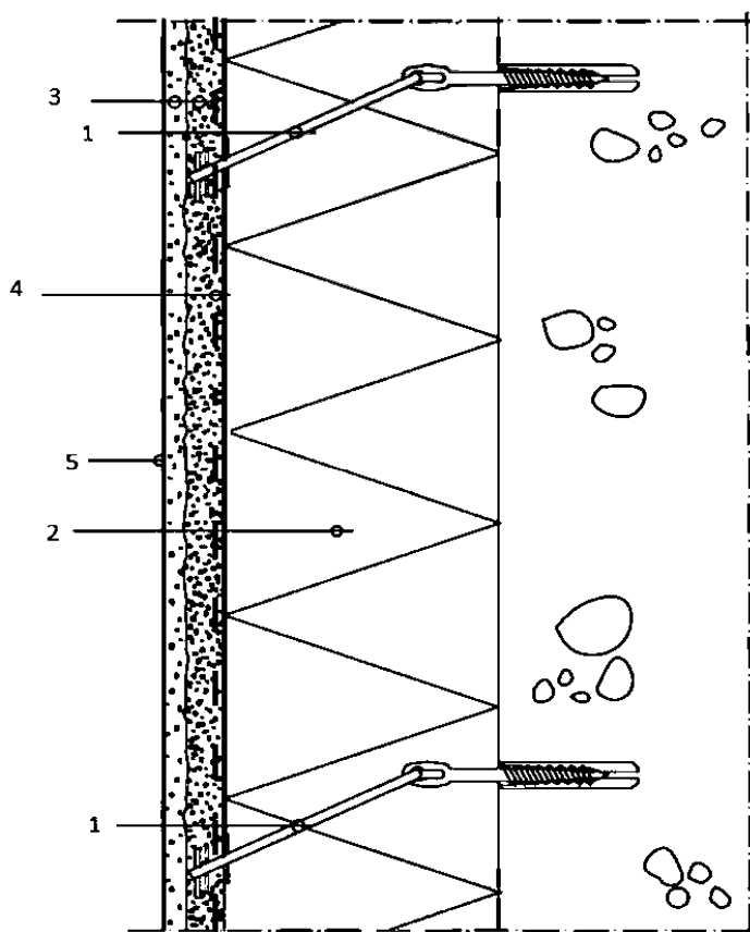
1 – шарнирный анкер; 2 – теплоизоляционный слой; 3 – штукатурный слой; 4 – армирующая сетка; 5 – декоративно-отделочный слой
