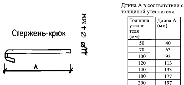
Рисунок 7 – Стержень-крюк шарнирного анкера
