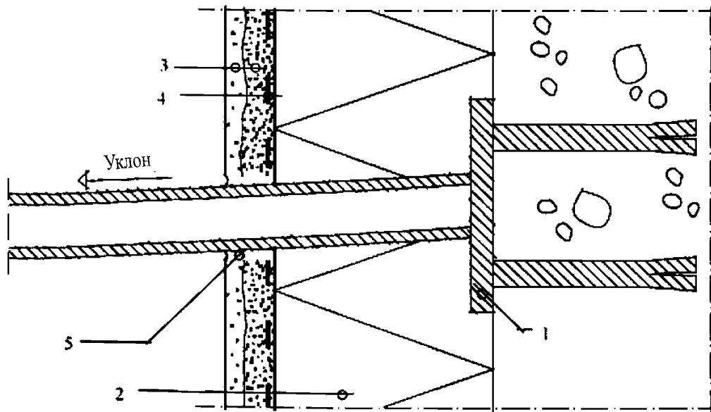
Рисунок 9.8 – Устройство системы в месте устройства воздуховодов
