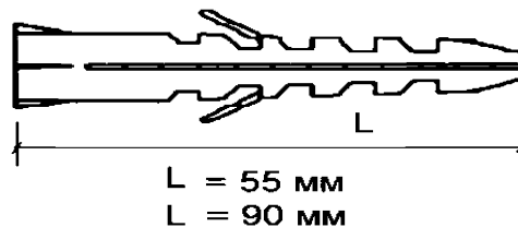
Рисунок 6 – Пластиковый дюбель шарнирного анкера
