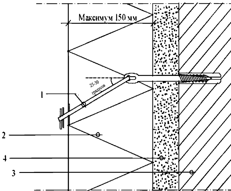
Рисунок 12 – Установка плит утеплителя в проектное положение
