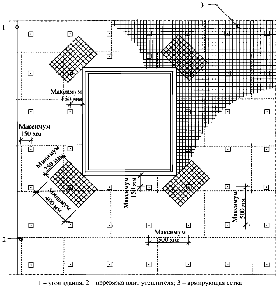
Рисунок 14 – Усиление вершин углов проемов в основании
