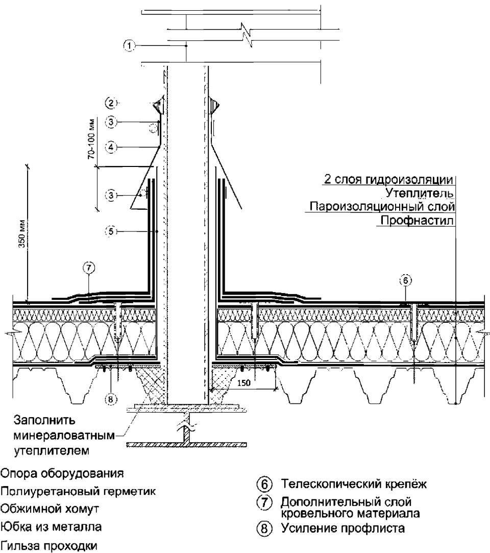
Рисунок 1 – Устройство примыкания к опоре с гильзой на плоской крыше
