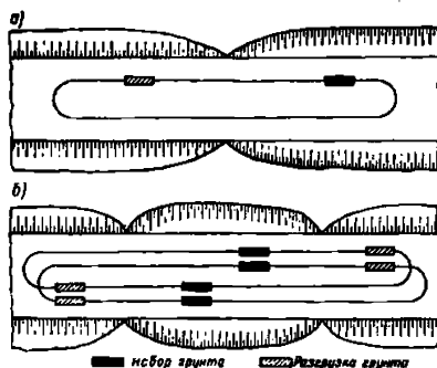
Рисунок 5 – Схема движения скрепера при разгрузке грунта в выемке с перемещением его в насыпь
